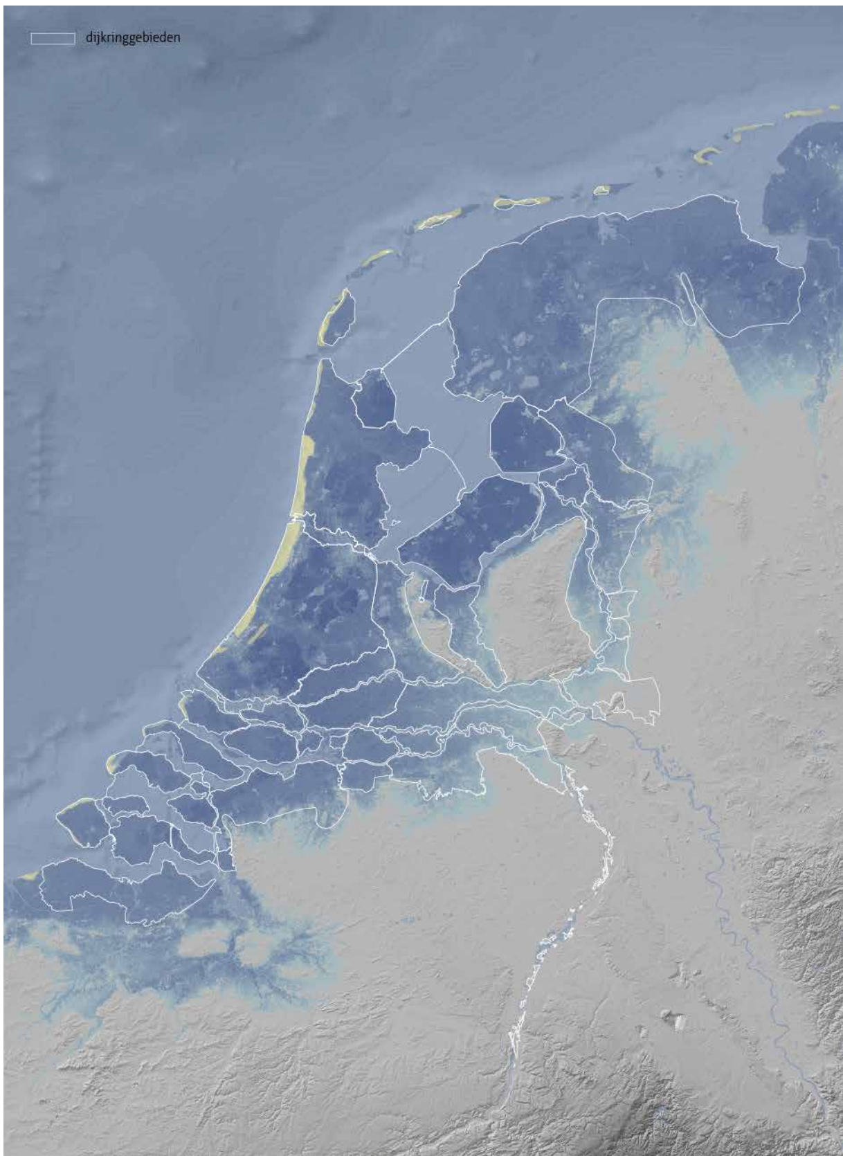
ILLUSTRATIE 3.6 Dijkkringgebiedenkaart in combinatie met de hoogtekaart.
