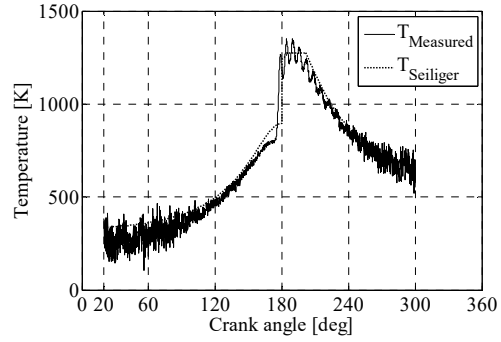
(d) Cylinder temperature (point B)
