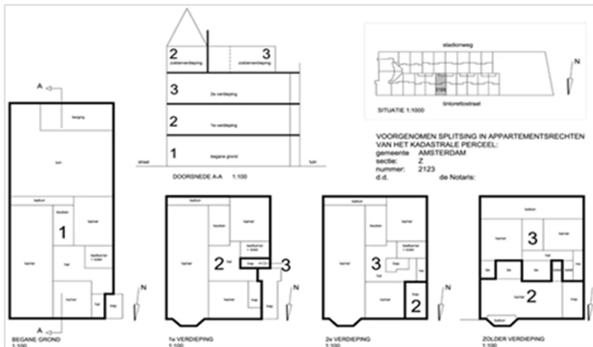
Fig. 1. A splitsingstekening (division drawing) (Max Architectuur BV, 2021).
