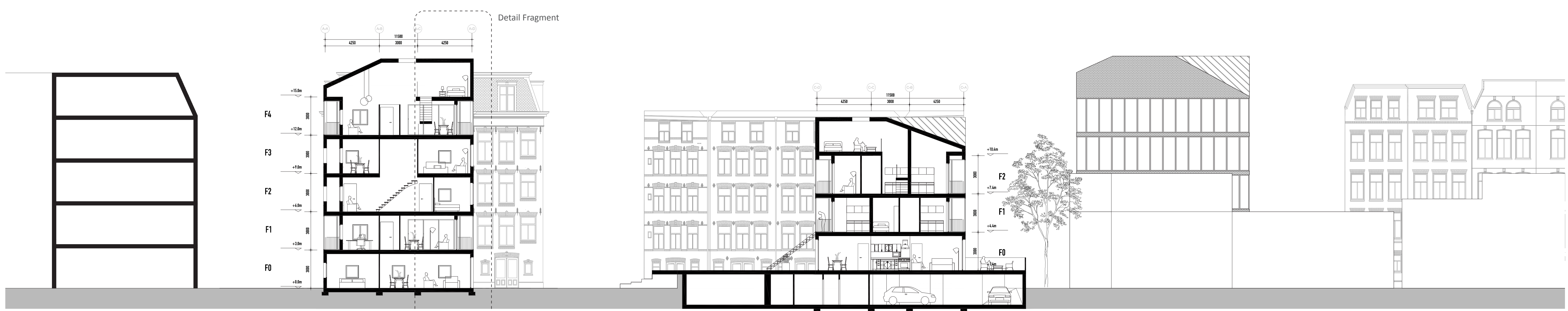
Section gg' 1:150
