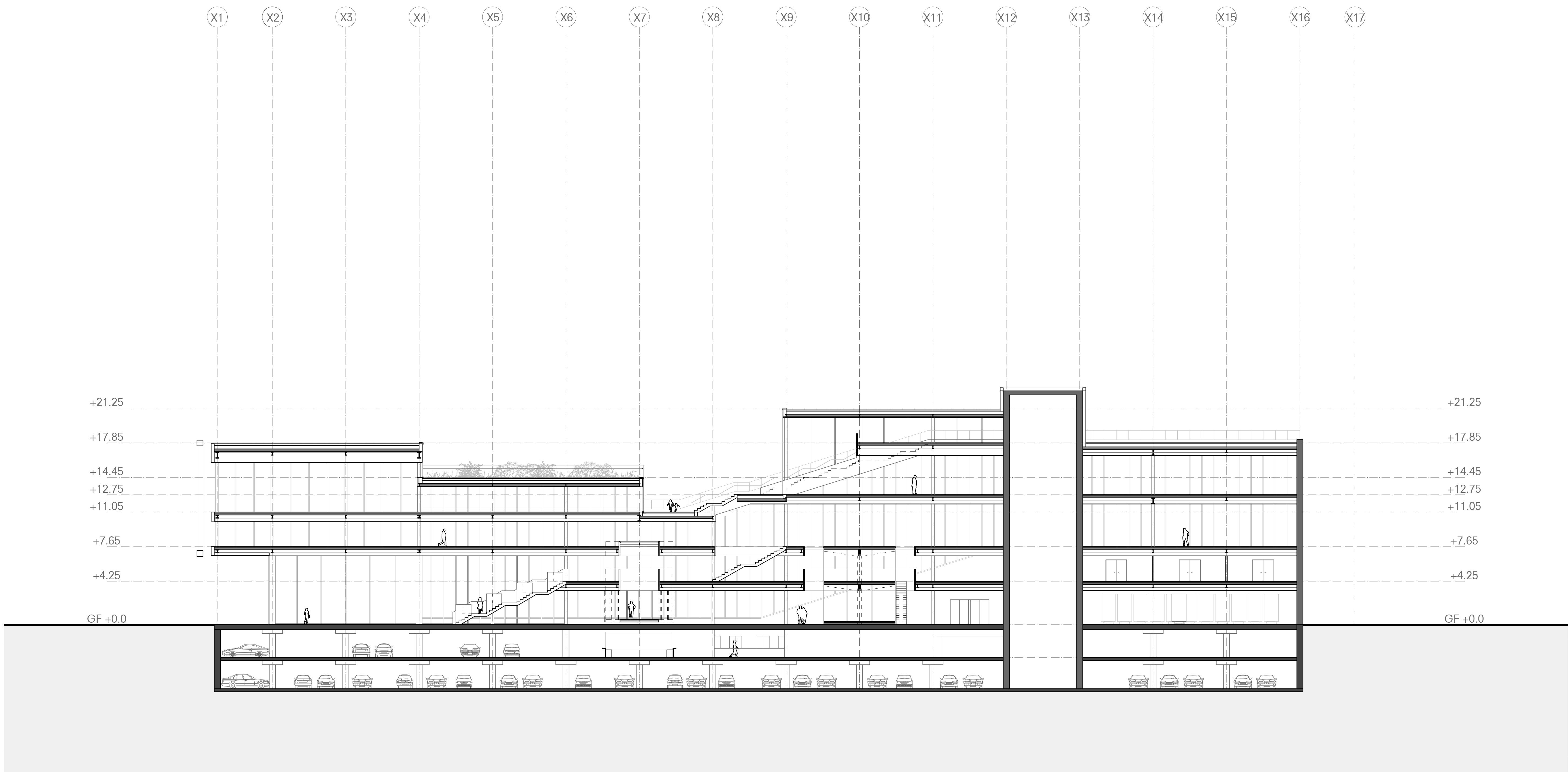
SECTION A-A 1:200
