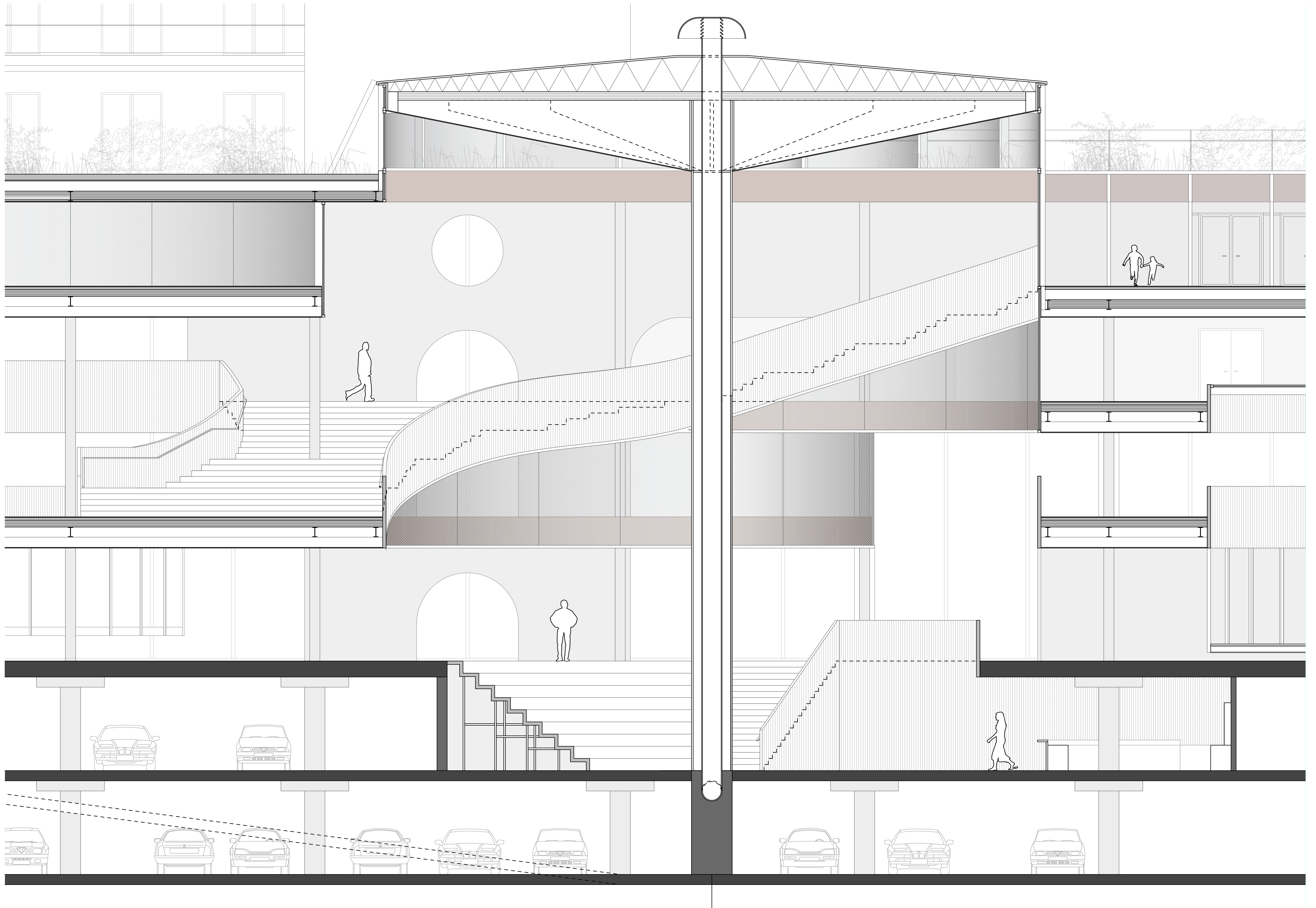
ATRIUM FRAGMENT 1:50
