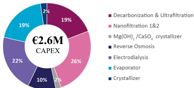
Fig. 8. Capital expenditure (CAPEX) for Bolesław Śmiały case.
