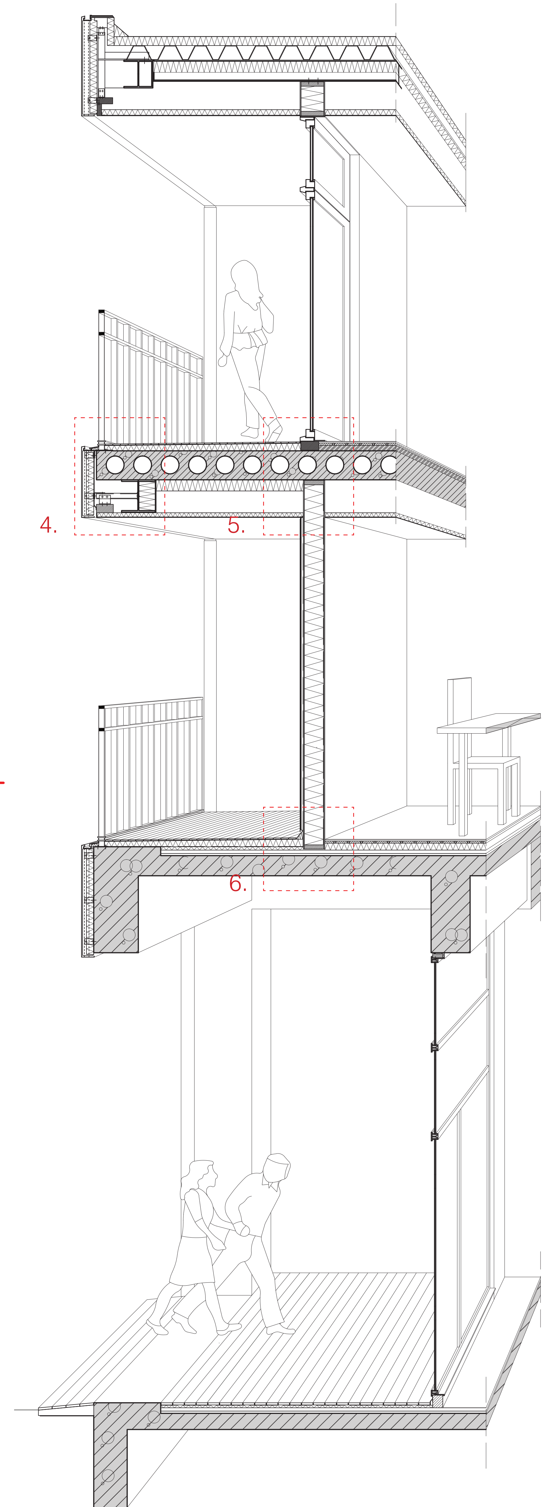
Verticale geveldoorsnede B 1:20
