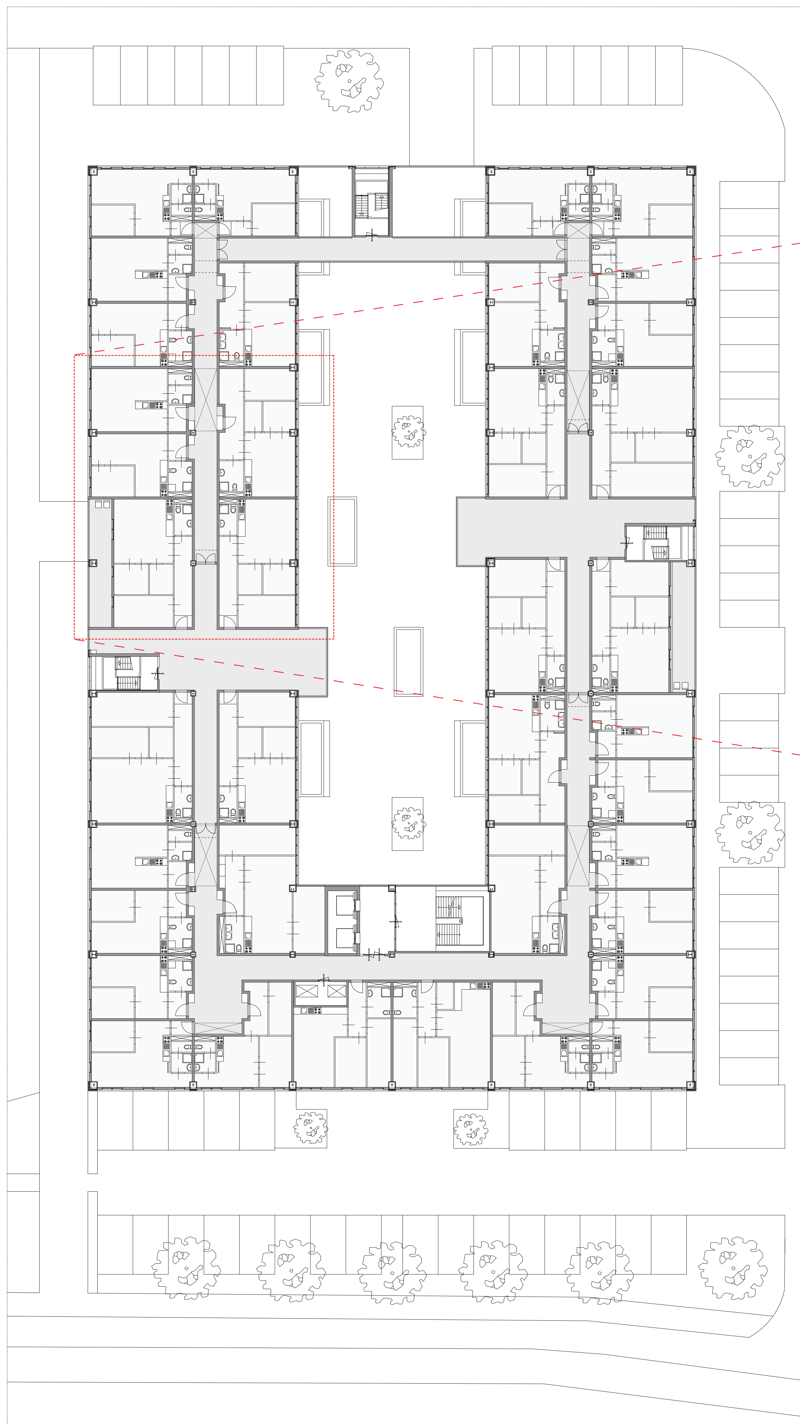
2e verdieping transformatieontwerp 1:200
