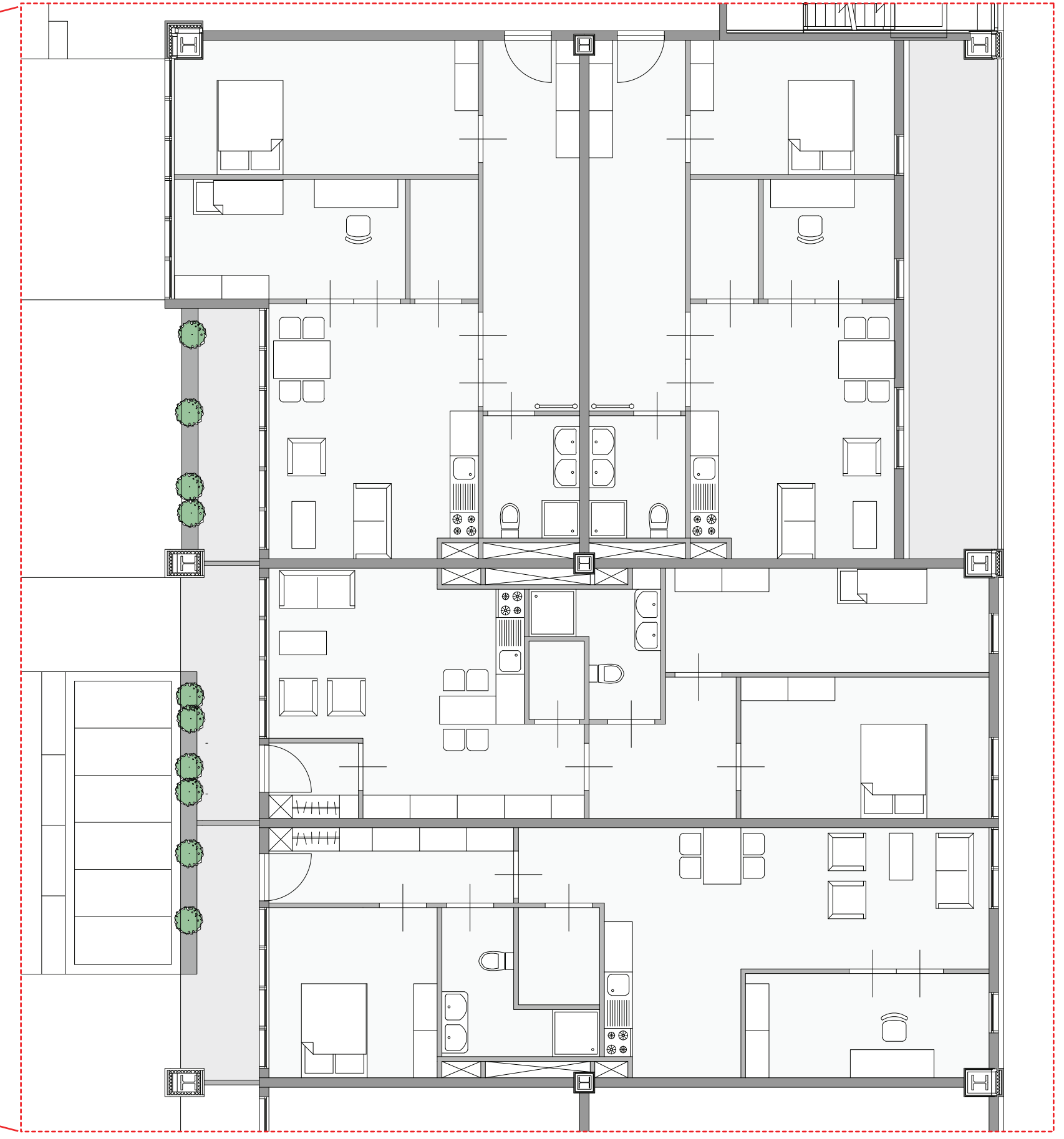
1e verdieping woningen jonge gezinnen 1:100
