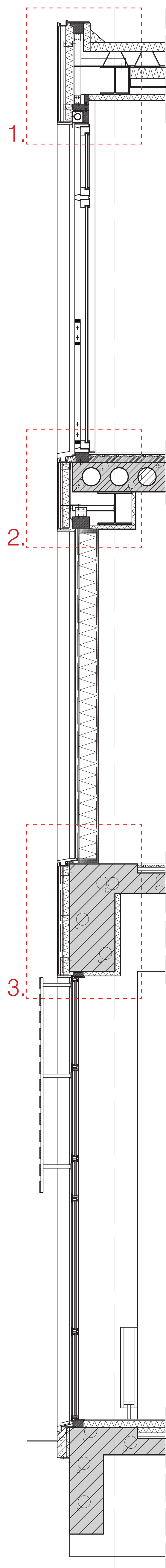
Verticale geveldoorsnede A 1:20
