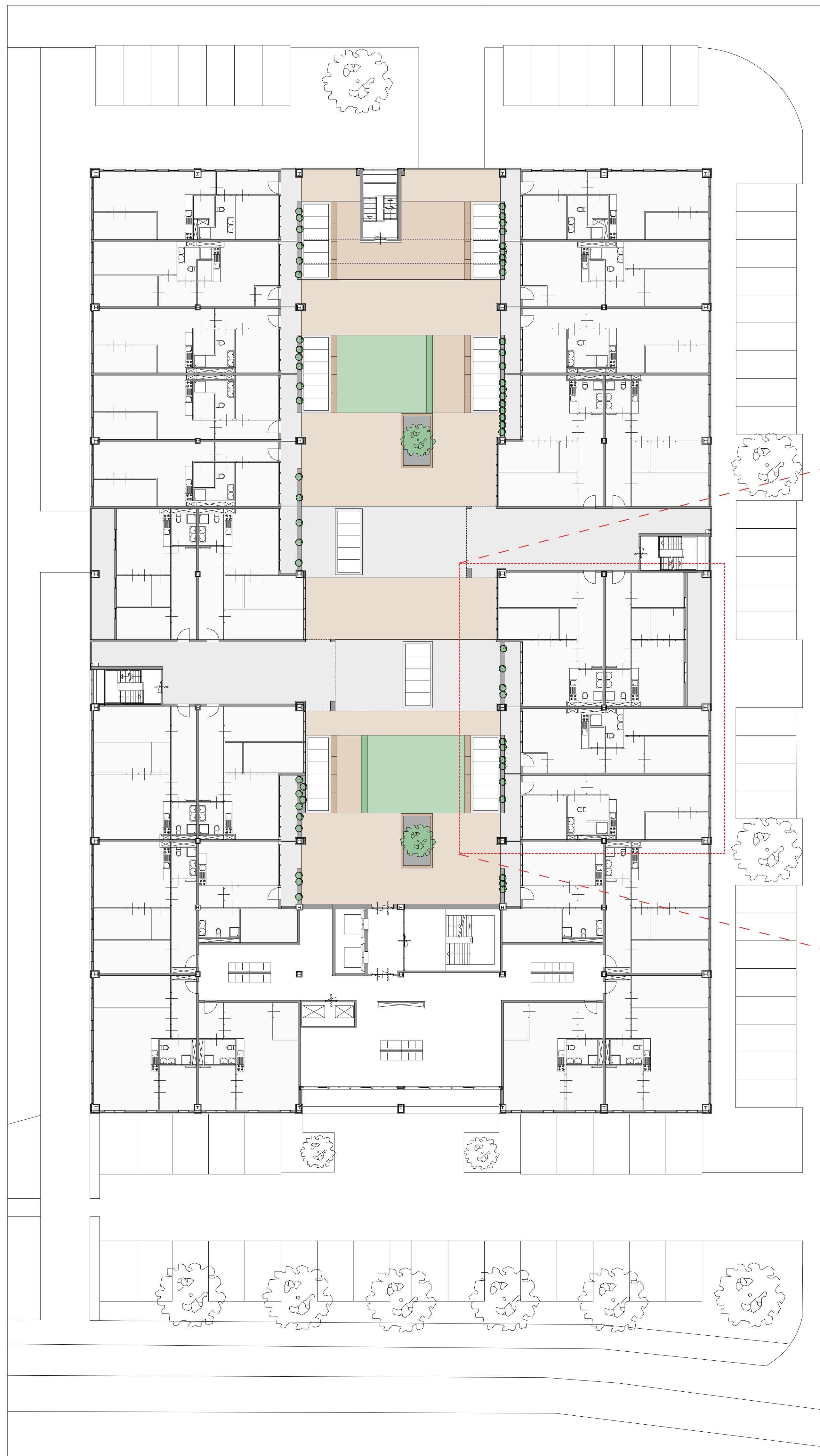
1e verdieping transformatieontwerp 1:200
