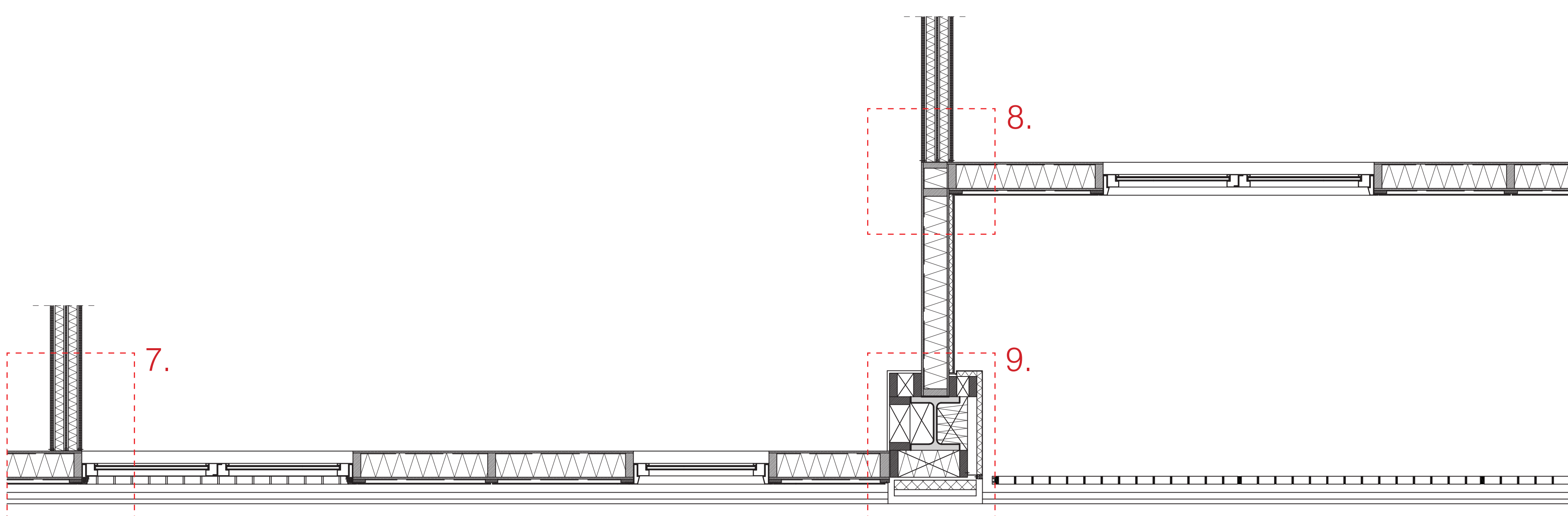
Horizontale geveldoorsnede 1:20
