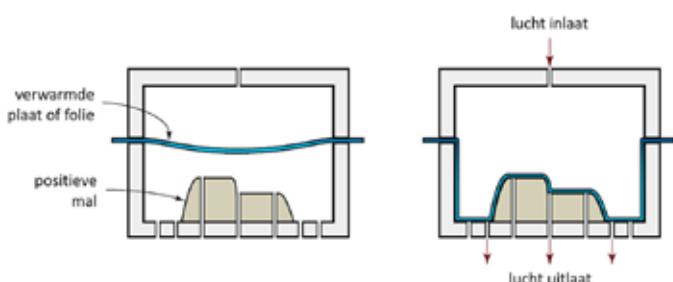
Afbeelding 4 Positief thermovormen
