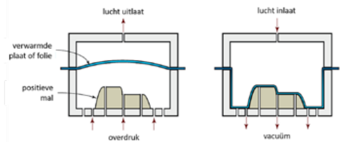
Afbeelding 5 Thermovormen met voorblazen
