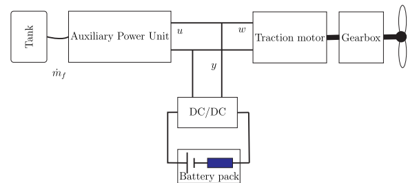
Fig. 1. Powertrain diagram
