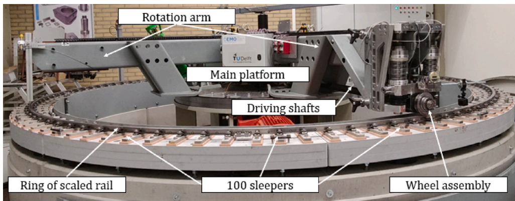
Fig. 1. The V-Track test rig.
