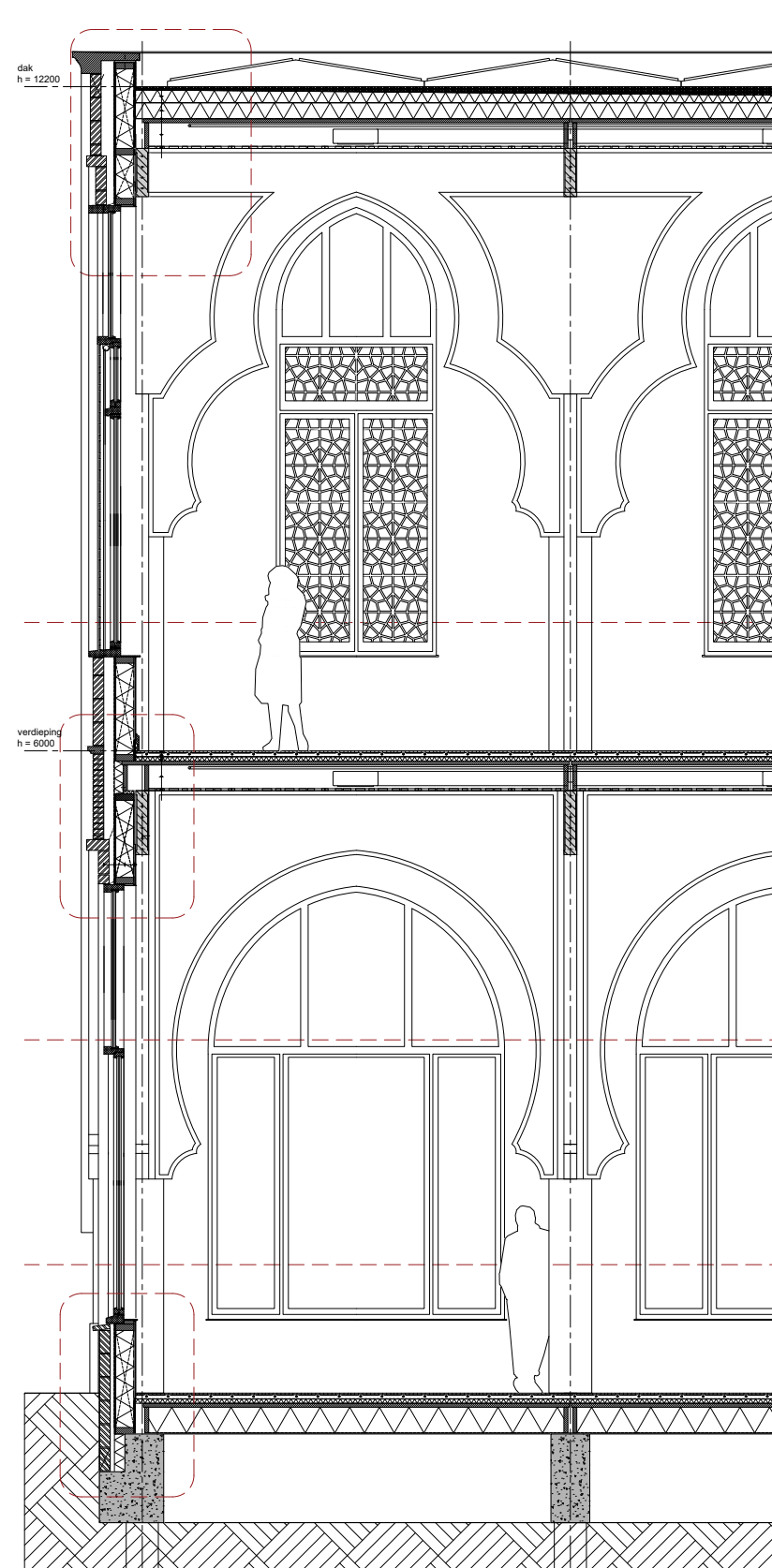
uitgewerkt gevelfragment gevelontwerp
