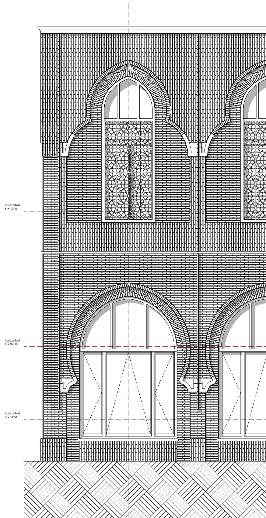
uitgewerkt gevelfragment gevelontwerp
