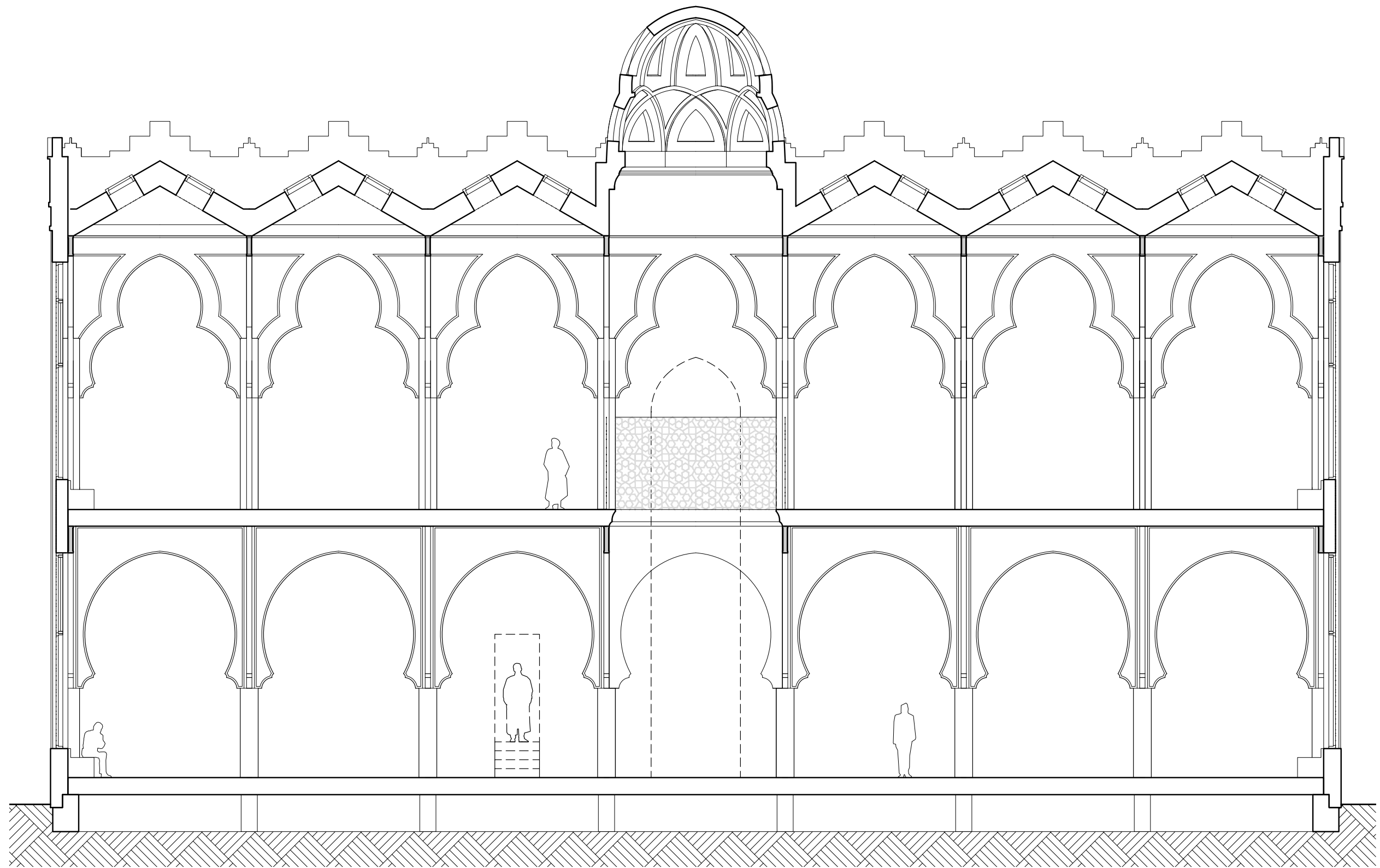
Doorsnede gebedshal scheiding man/vrouw
