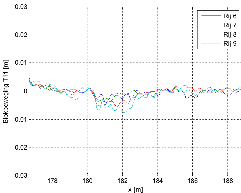
Figuur C.7b Niveau van het taludoppervlak over dwarsprofielen 6-9 (Proef 11)
