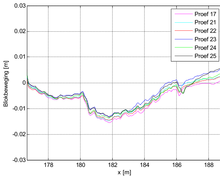
Gemiddelde niveau van het taludoppervlak over dwarsprofielen 5-9, waarin geen kabel in het profiel voorkomt.
