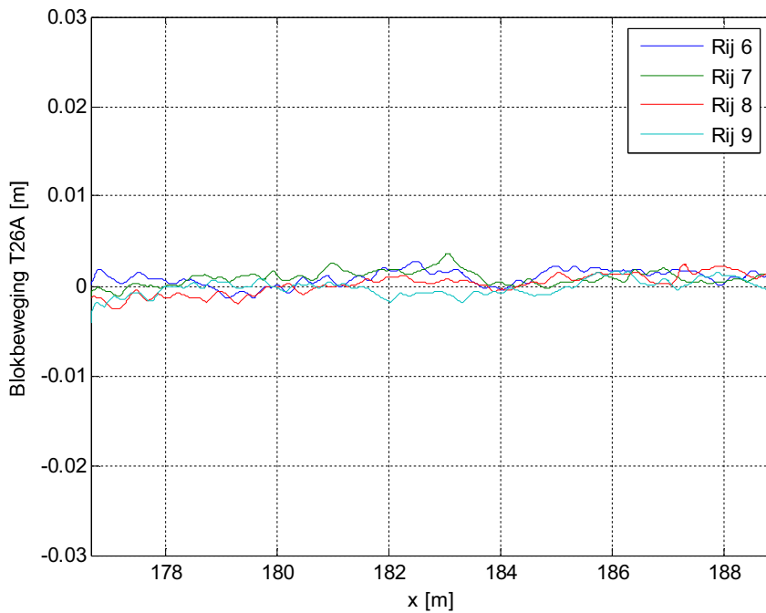
Figuur C.20b Niveau van het taludoppervlak over dwarsprofielen 6-9 (Proef 26A)
