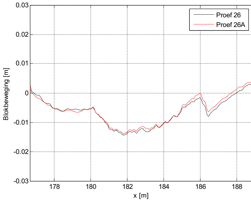
Figuur C.3a Gemiddeld niveau van het taludoppervlak over dwarsprofielen 5-9, zonder versterking door de kabel op blokrij Z (Proef 26)
