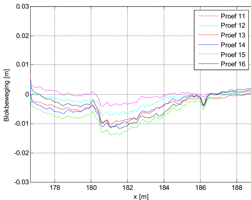
Figuur C.1a Gemiddeld niveau van het taludoppervlak over dwarsprofielen 5-9, zonder verstoring door de kabel op blokrij Z (Proef 11-16)
