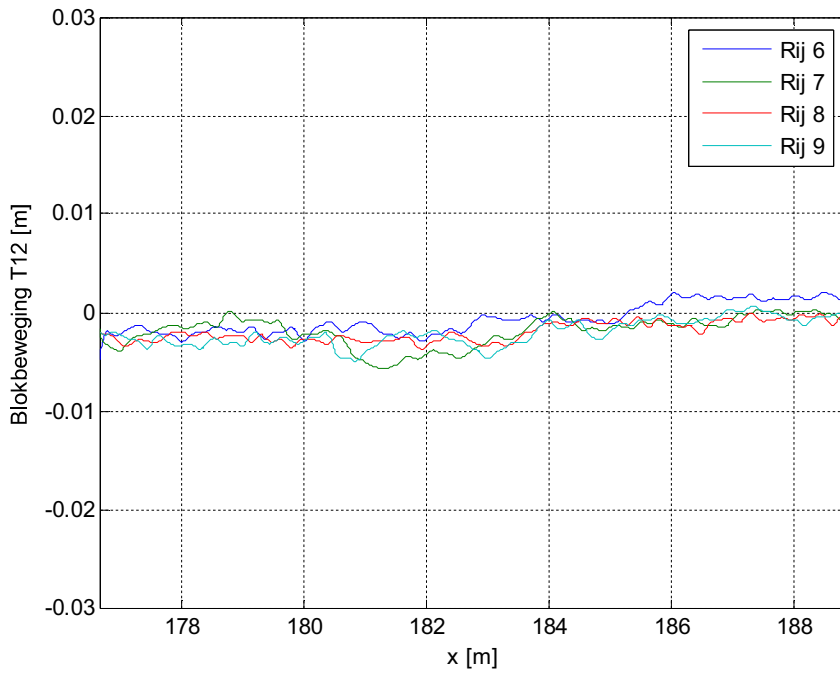
Figuur C.8b Niveau van het taludoppervlak over dwarsprofielen 6-9 (Proef 12)
