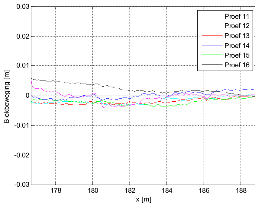
Figuur C.4a Gemiddeld niveau van het taludoppervlak over dwarsprofielen 5-9, zonder verstoring door de kabel op blokrij Z (Proef 11-16)
