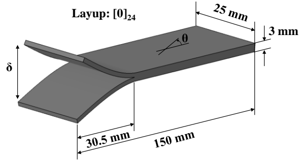
Fig. 5 DCB specimen.
