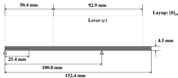
Fig. 8 MMB specimen.
