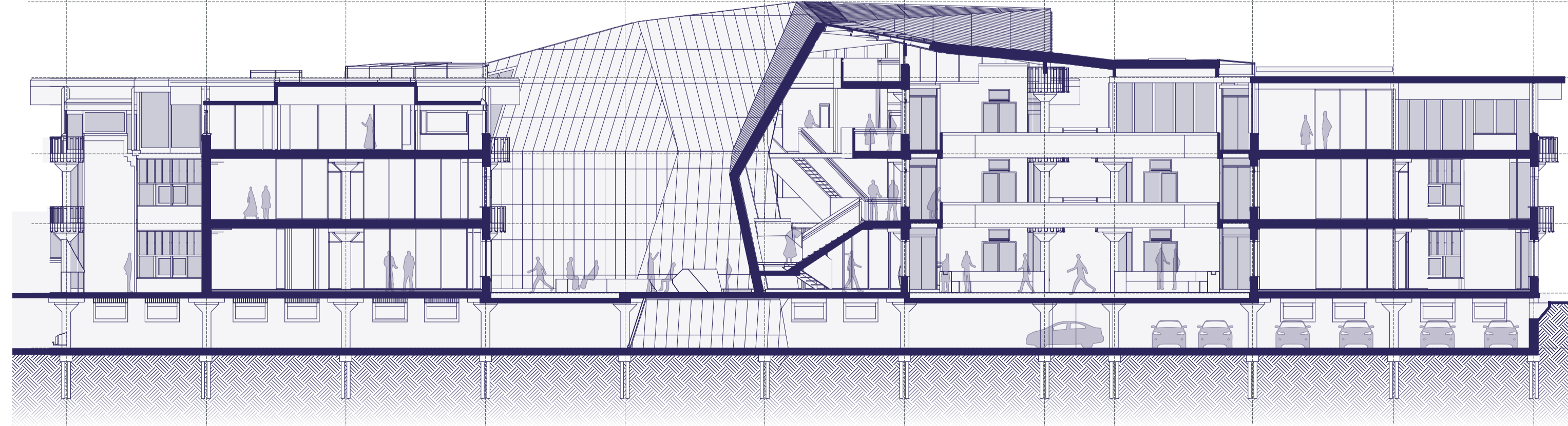
SECTION D-D' // 1:200
