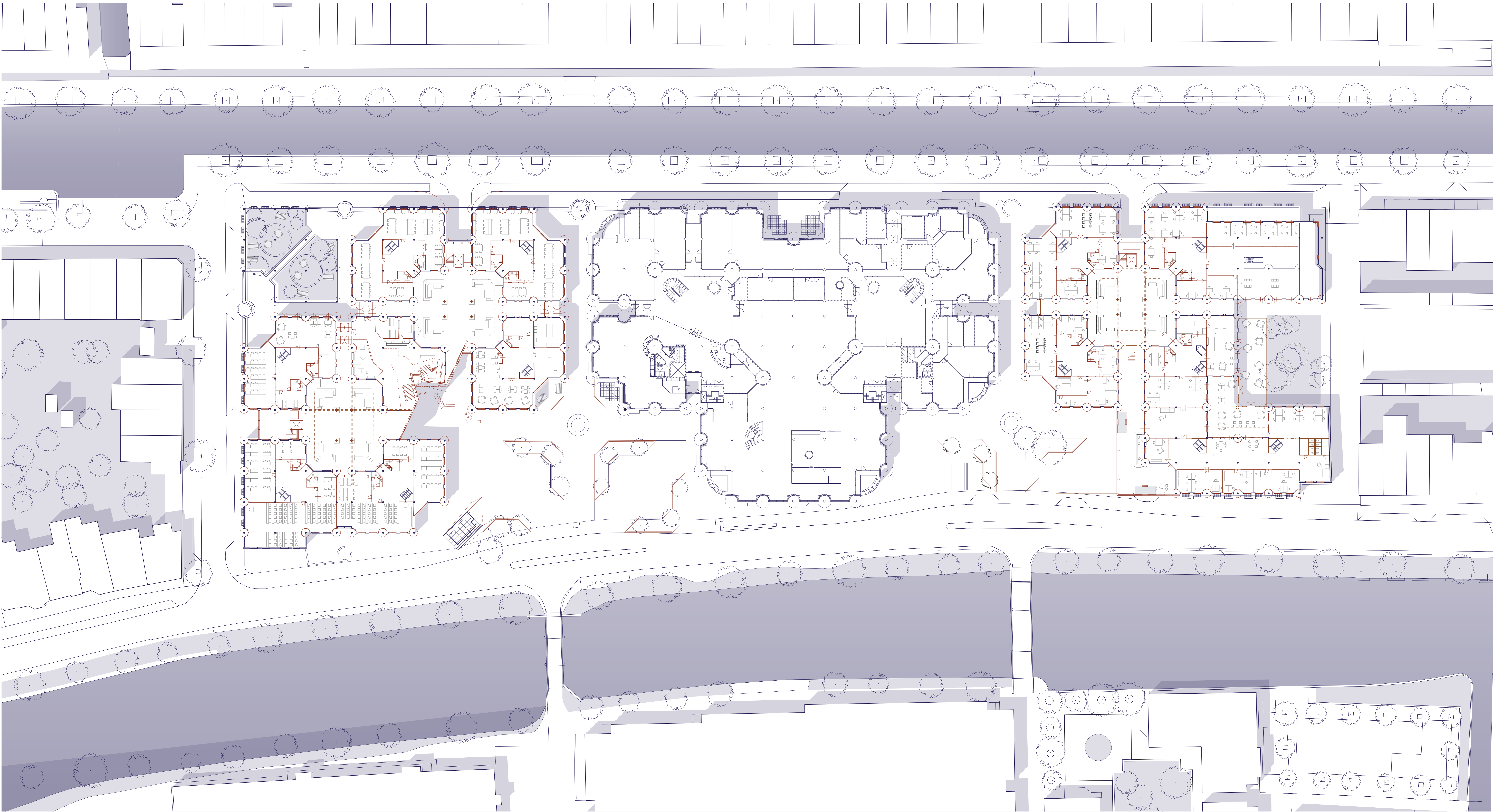
SITUATION PLAN // 1:300
