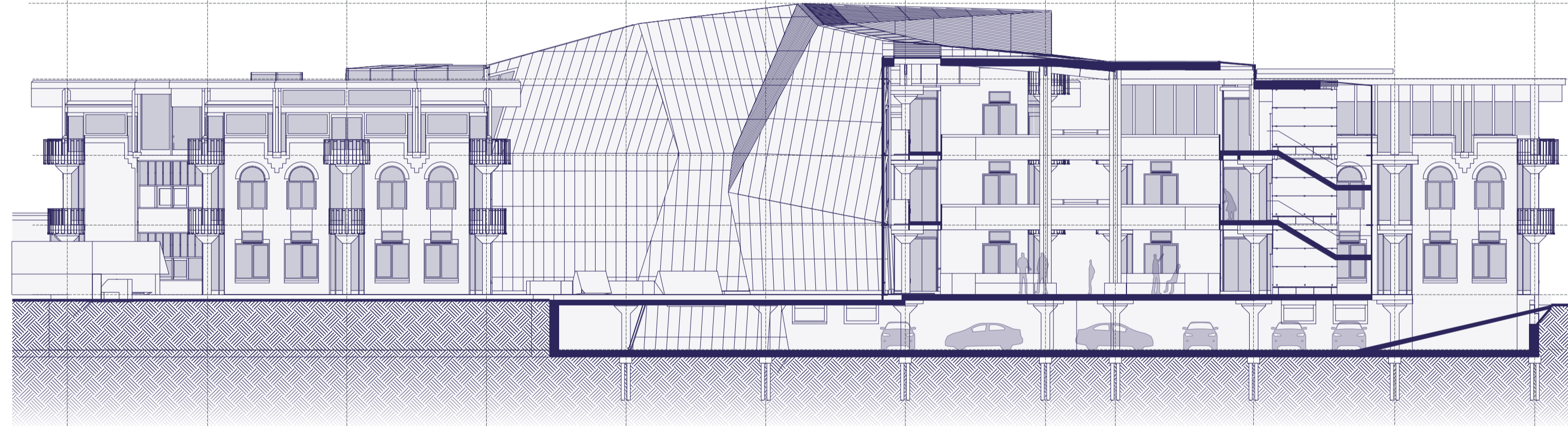
SECTION C-C' // 1:200
