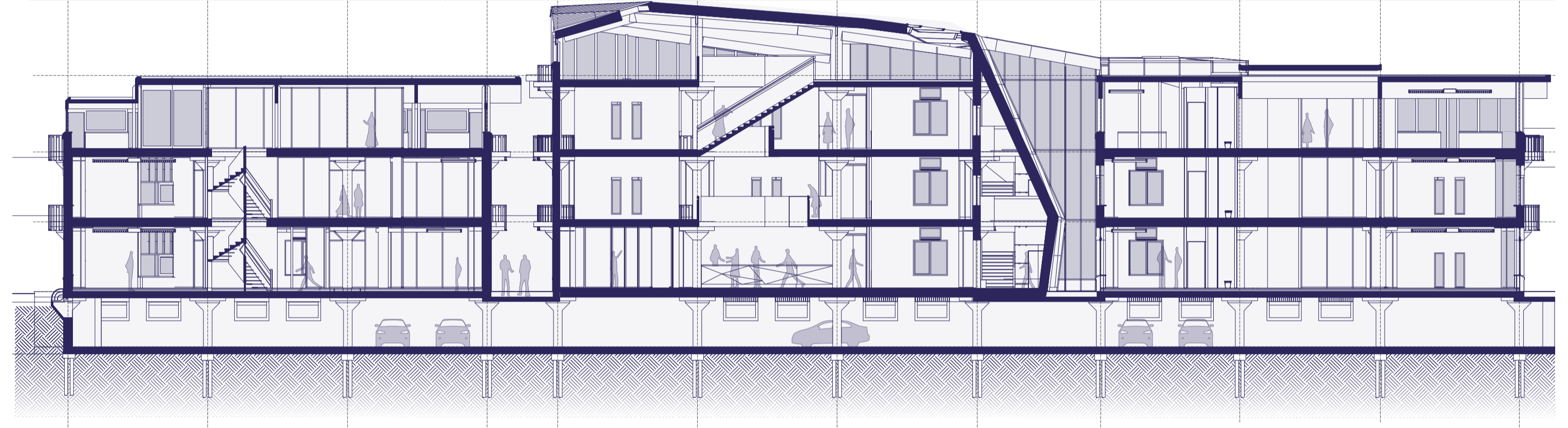
SECTION B-B' // 1:200
