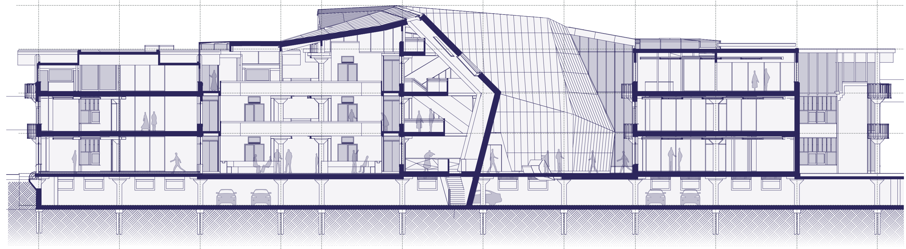
SECTION A-A' // 1:200
