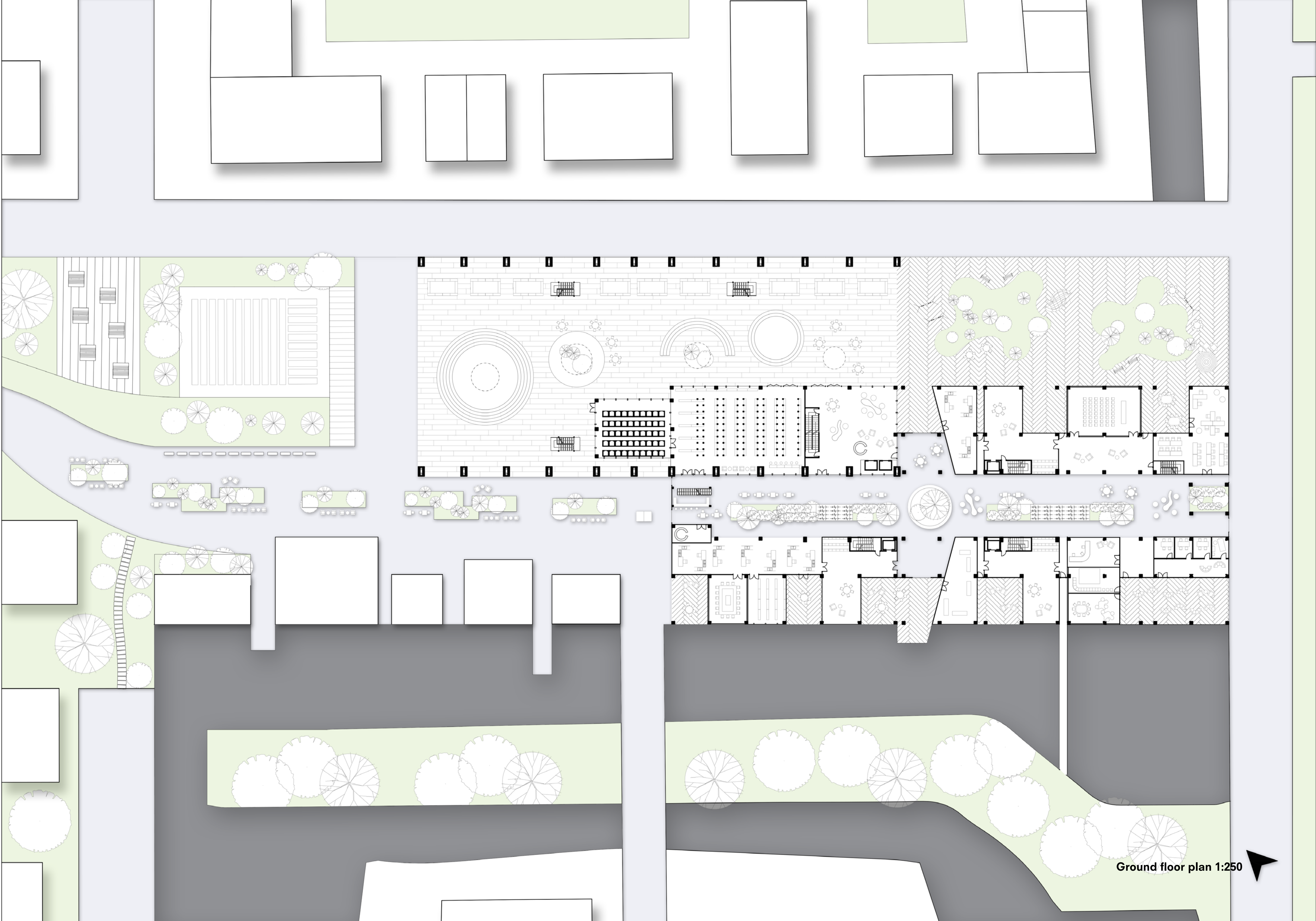
Site plan 1:1000
