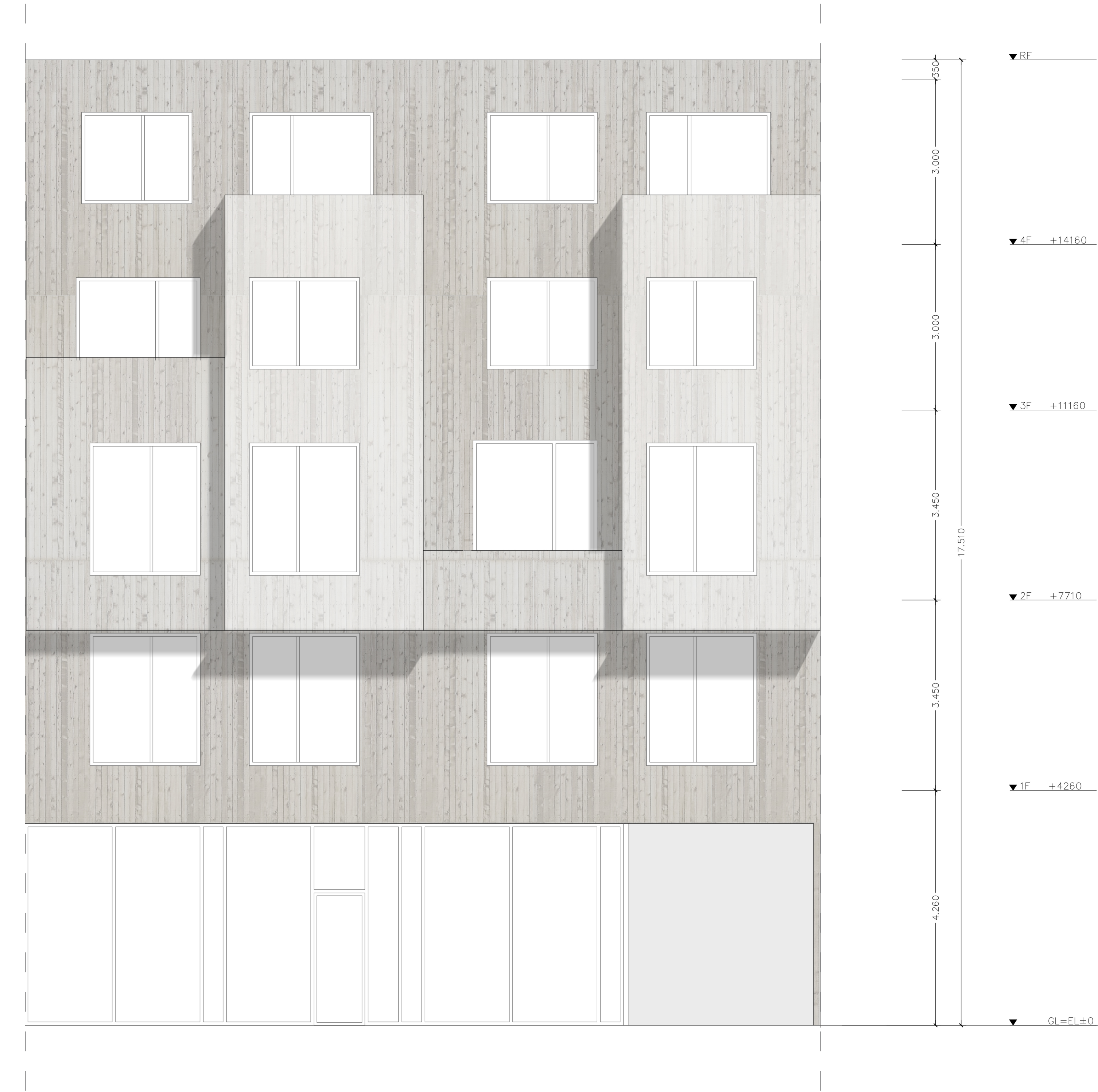
Elevation 1:50
