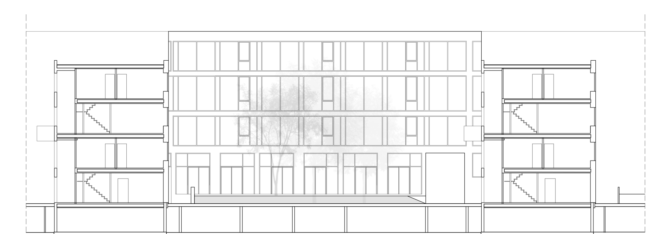
BB Section 1:200
