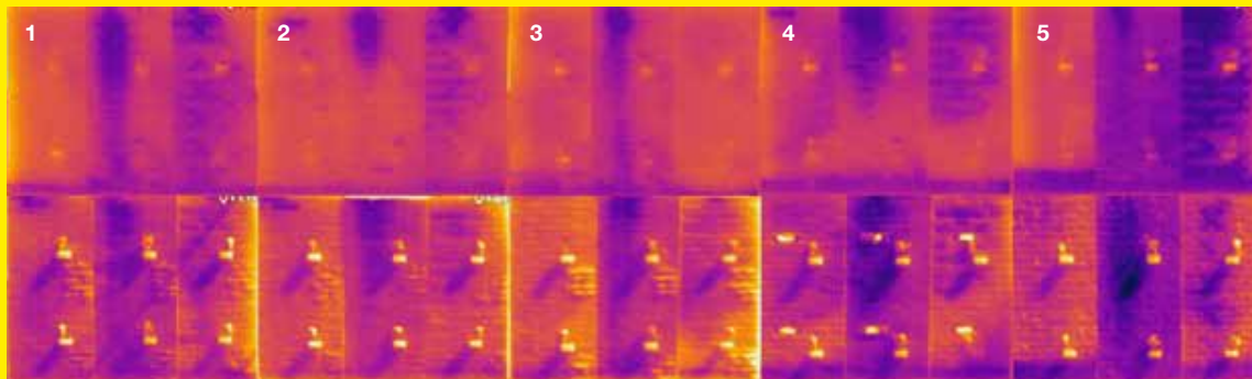
Thermobeeld van de panelen gericht op NNO (boven) en ZZW (onder). De blauwe delen zijn het koelst. Foto's gemaakt op een warme dag na drie dagen droogte. 23 juni 2020, rond 10:30 uur.
