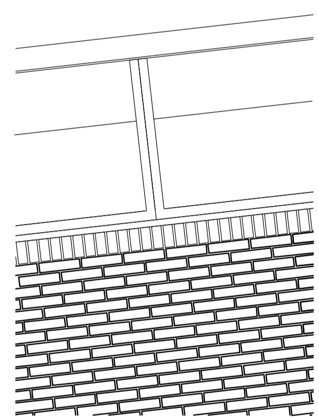
Exterior 1:20
