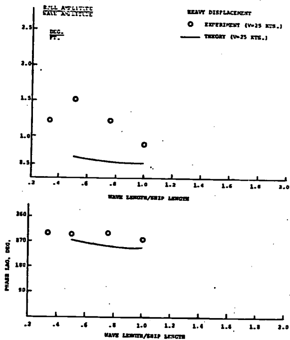
Fig. 8 - Roll & Phase Lag, 60° Heading
