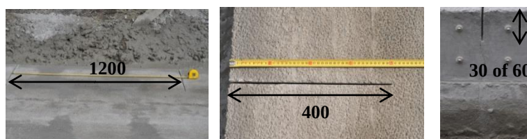
Figuur 10. Onderlinge afstand (links), lengte (midden) en diepte (rechts) van de korte dwarse zaagsneden in de proefvakken op de E313 bij Herentals; dimensies in mm.
