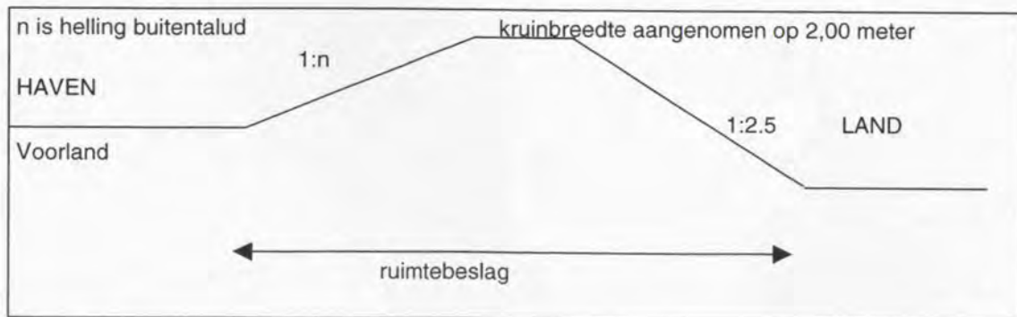
figuur 4: definitieschets
