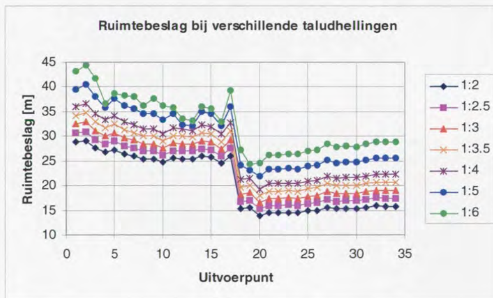
Figuur 6: Ruimtebeslag bij glad talud
