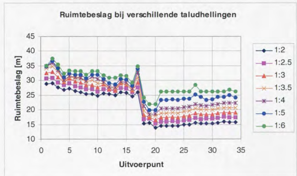
Figuur 13: Ruimtebeslag bij talud met berm
