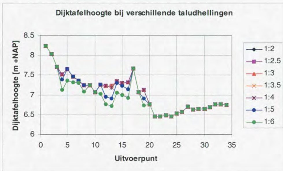
Figuur 5: Dijktafelhoogte bij glad talud
