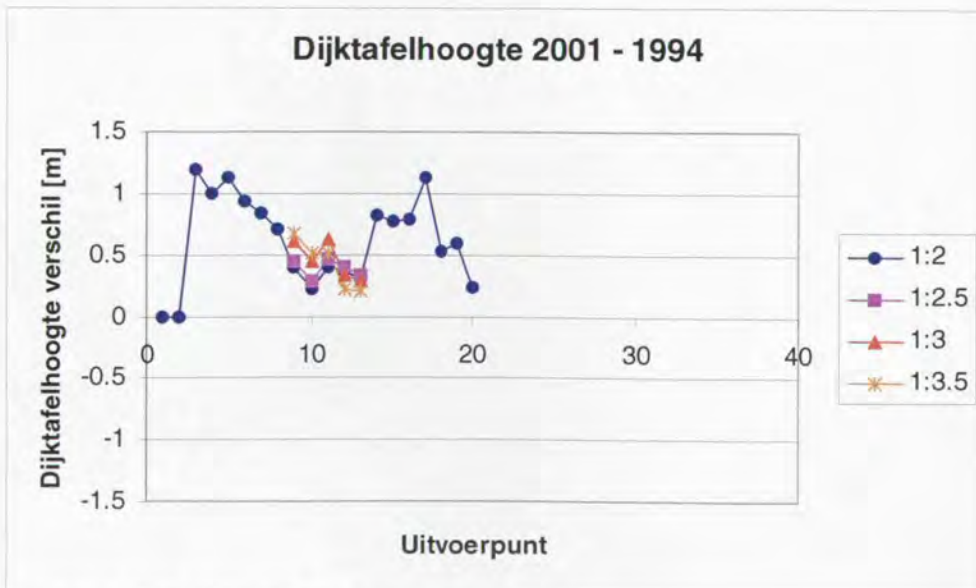
Figuur 15: Dijktafelhoogte verschil bij talud met berm
