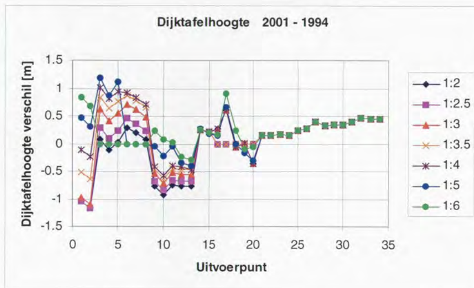
Figuur 7: Verskil in kruinhoogte bij glad talud
