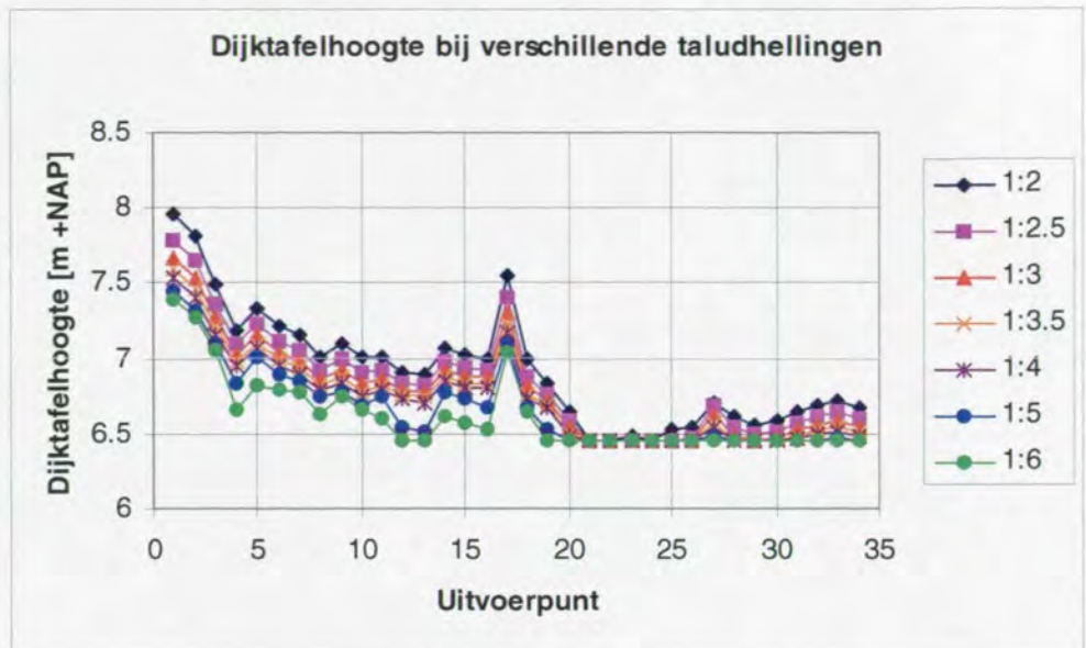
Figuur 8: Dijktafelhoogte bij ruw talud
