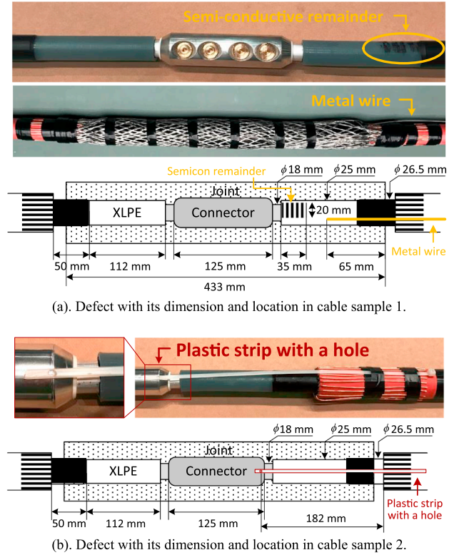
Fig. 4. Cable samples.
