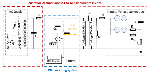
Fig. 3. Test circuit.
