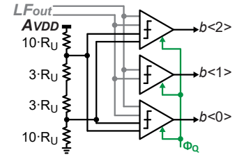
Fig. 4: 2b Flash quantizer
