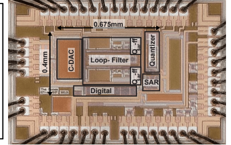
Fig. 5: Die micrograph
