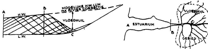
Fig. 7 Verklaring van het begrip vloedkuil.
