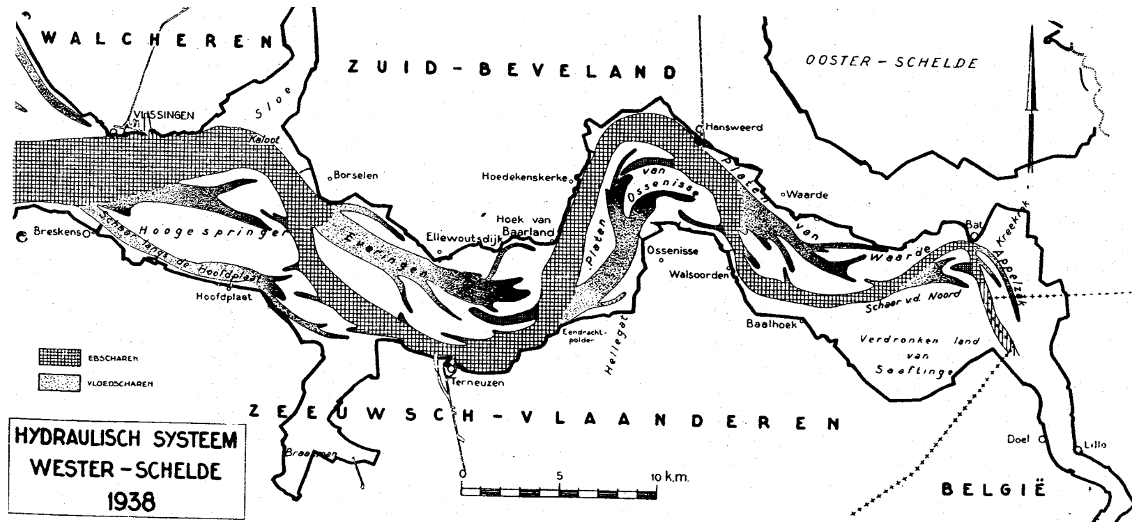
Fig. 28 System van eb- en vloedcharen op de Wester-Schelde in 1938.
