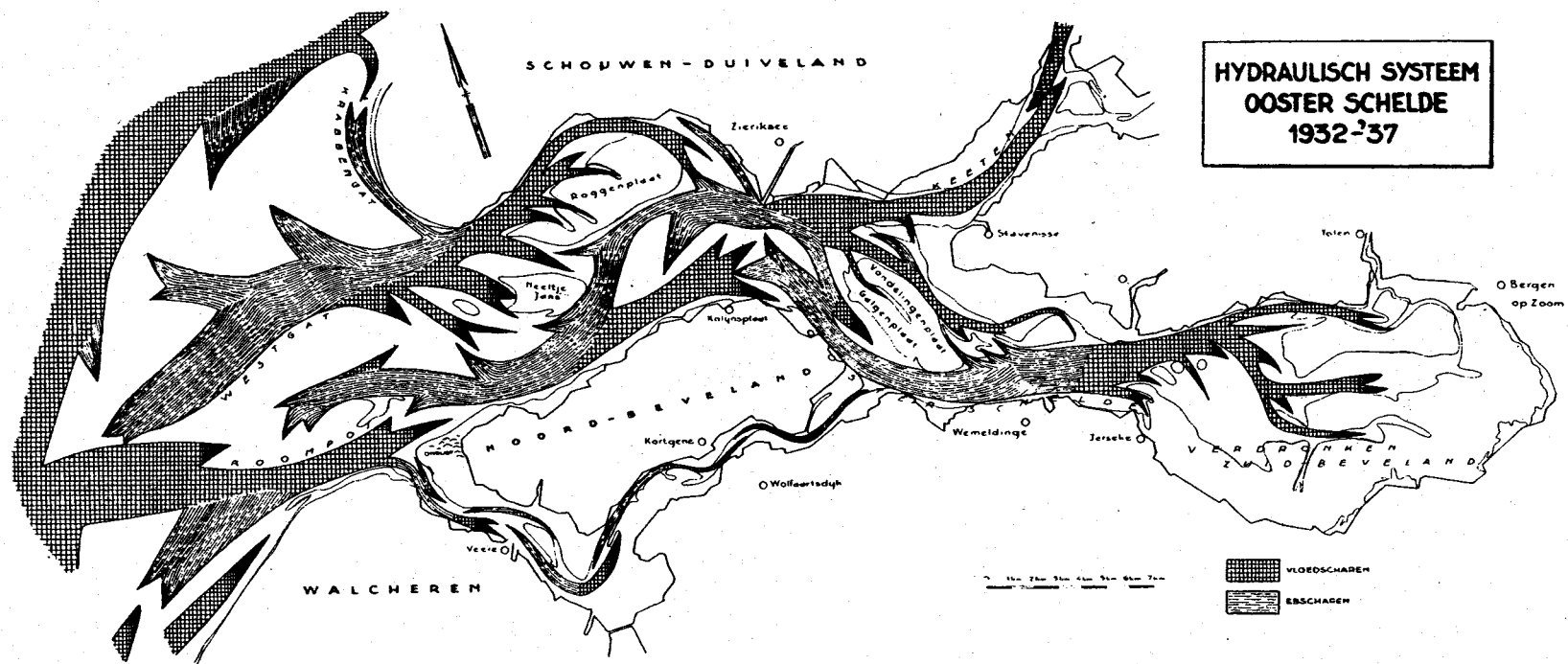
Fig. 29 System van eb- en vloedscharen op de Ooster-Schelde in 1937.
