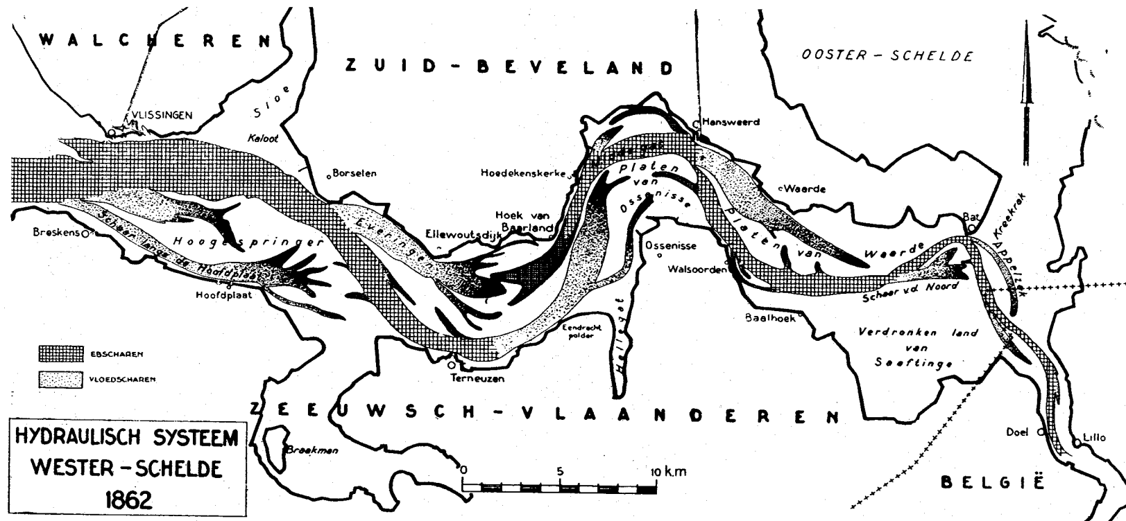
Fig. 27 System van eb- en vloedscharen op de Wester-Schelde in 1862.
