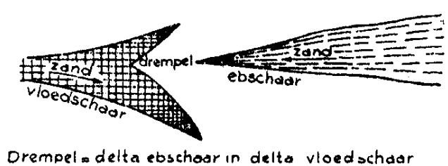
Fig. 10 Schema van het elkaar vermijden van een eb- en een vloodschar door middel van vorkvorming.
