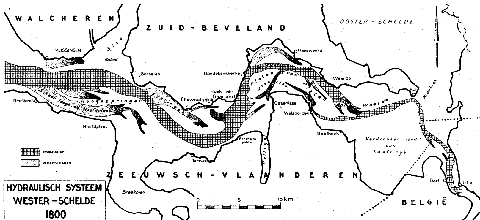
Fig. 26 System van eb- en vloedscharen op de Wester-Schelde in 1800.
