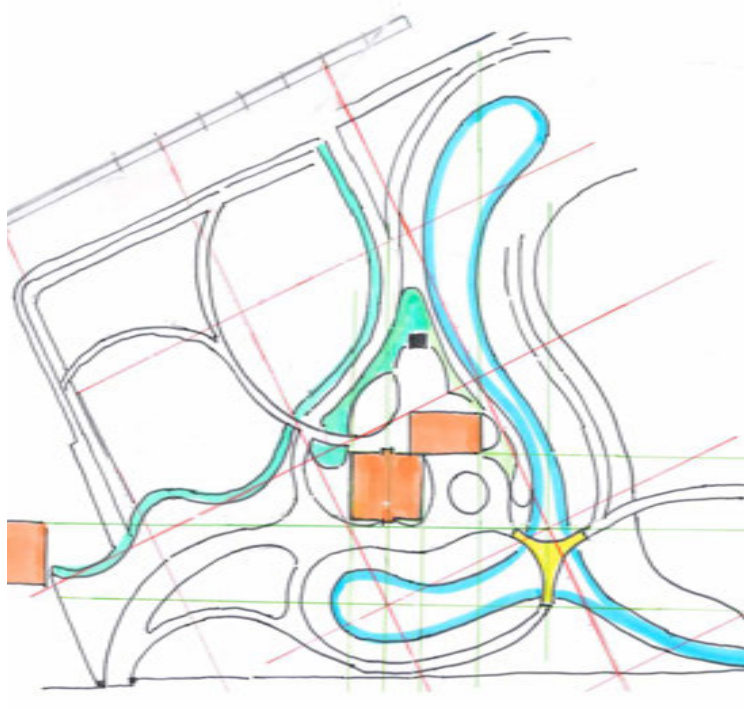
FIG. 6.4 Grafische vormgeving van structuurelementen met het maatraster, geconstrueerd vanuit de schaalbalk van het ontwerp voor de Grietenijtuin te Wolvega (Bron: auteur).
