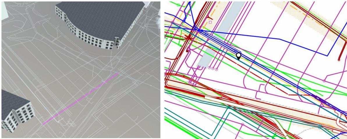
FIGUUR 6: TE VERVANGEN RIOOLBUIS IN DE 3D SITUATIE (LINKS - PAARS) EN IN DE 2D SITUATIE (RECHTS-GEMARKEERD)
