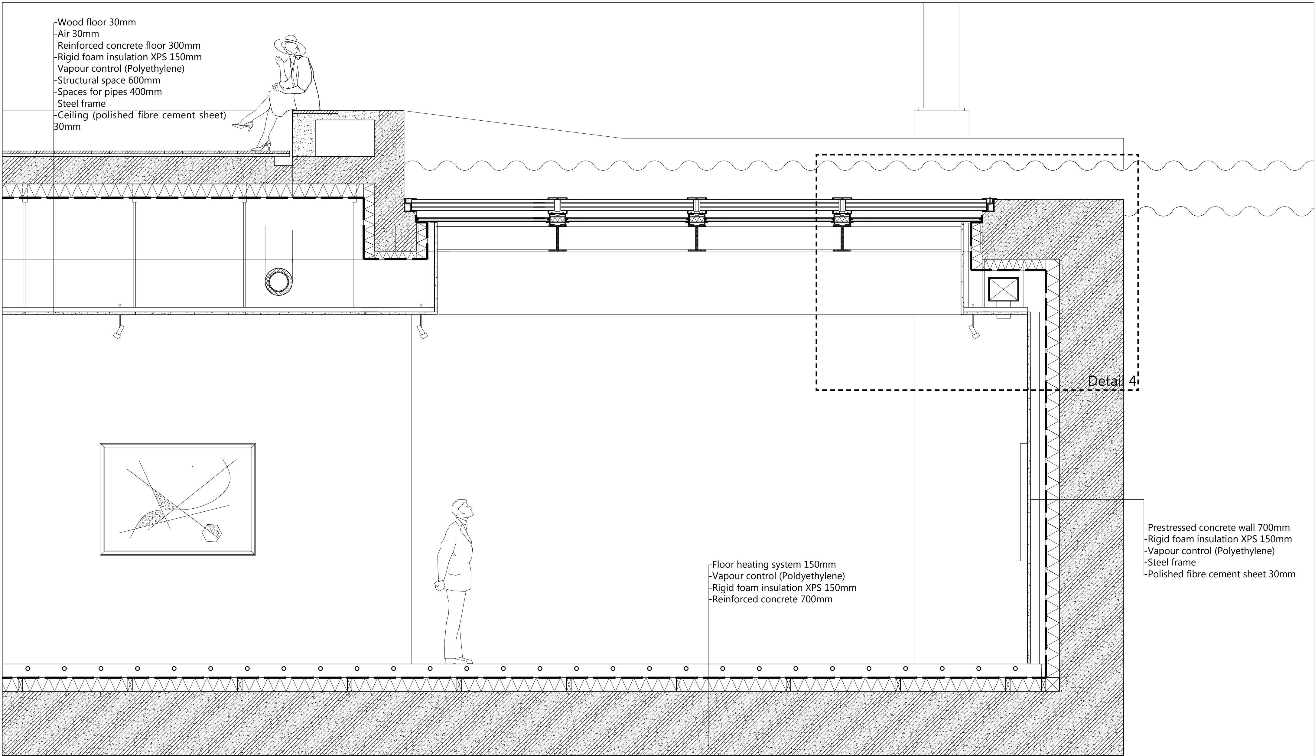
Section 4 1:25
