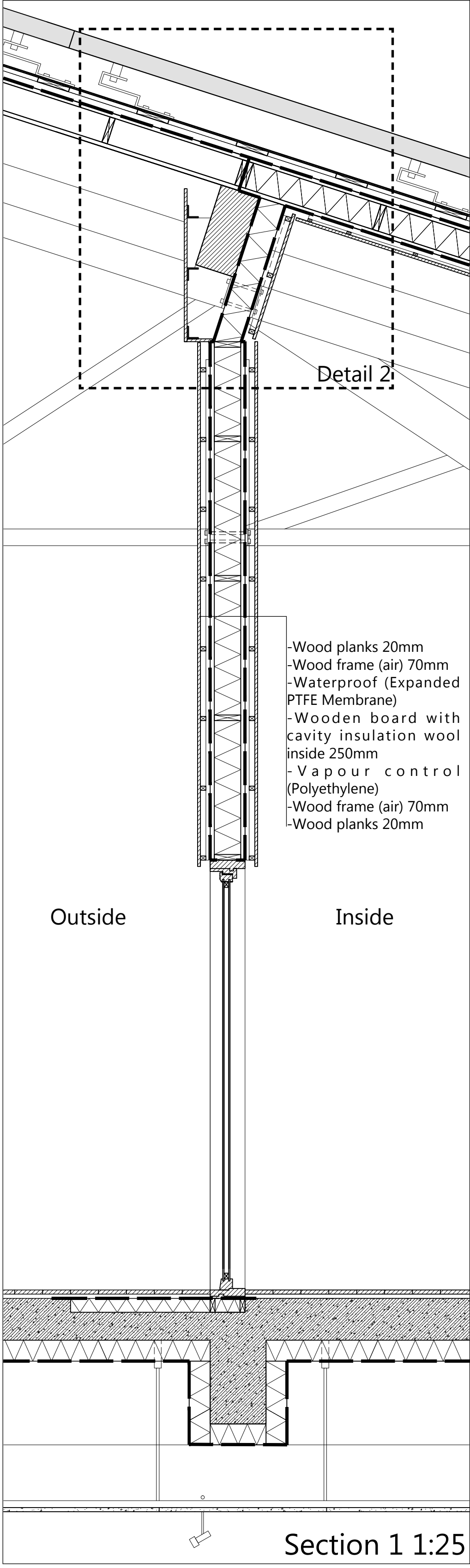
Section 1 1:25
