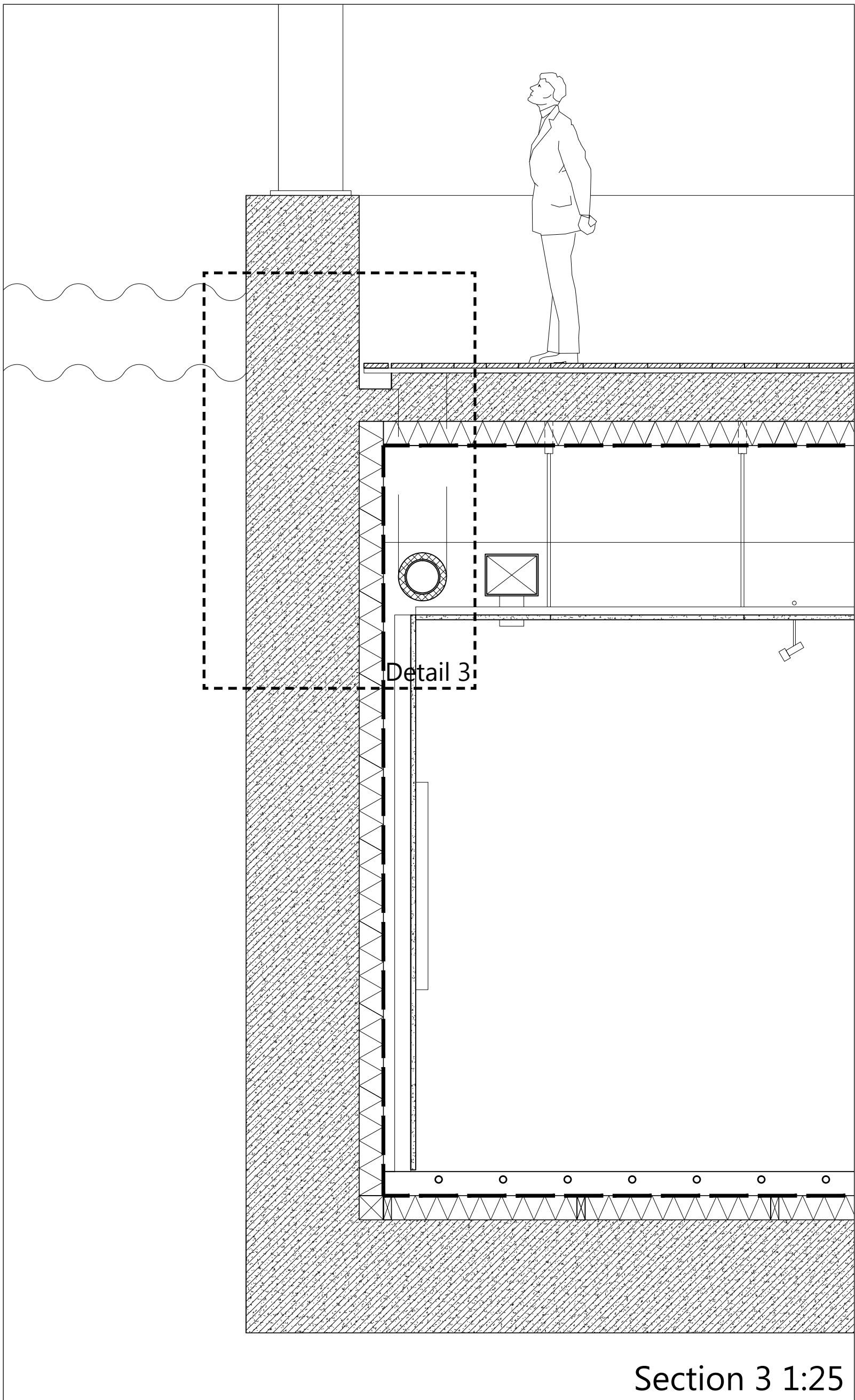
Section 3 1:25
