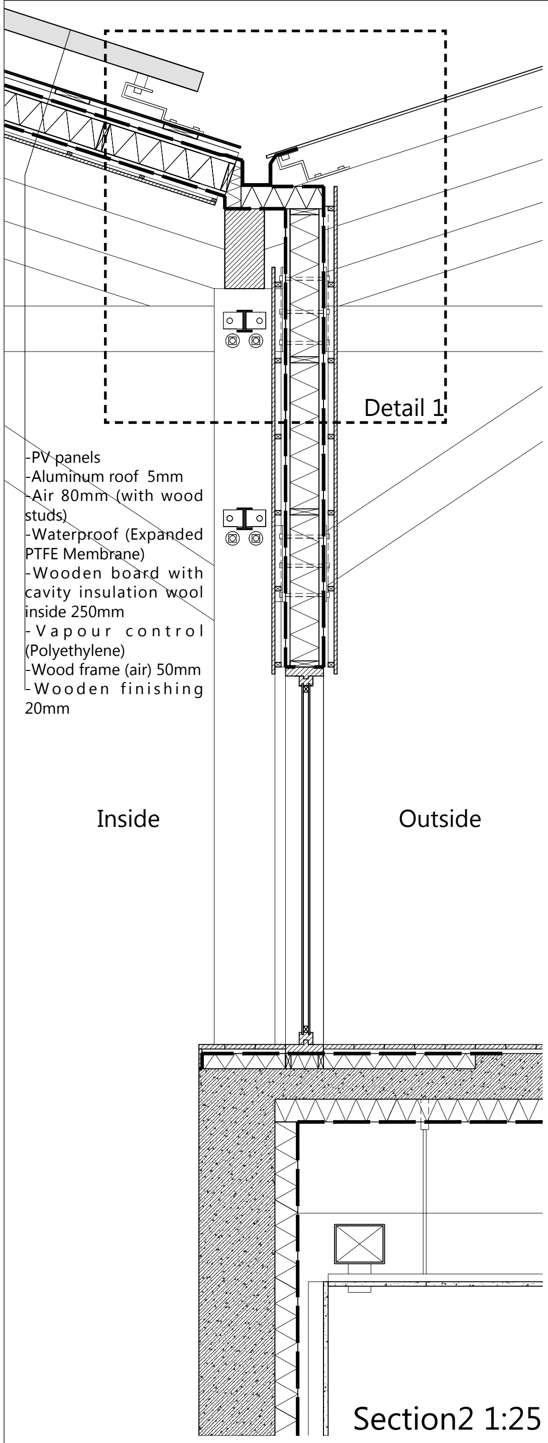
Section2 1:25
