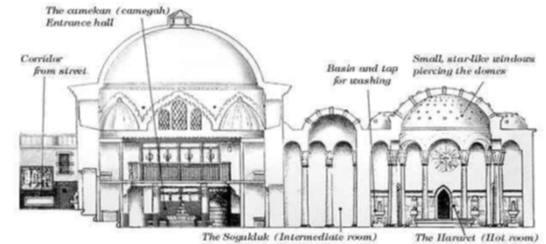
Doorsnede van de Cağaloğlu/Hamamı in Istanboel
