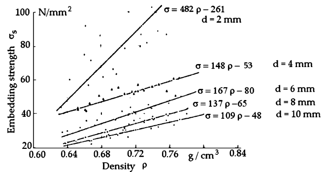
Fig. 2 Embedding strength dependent on the density; a = 19 \text{ mm} Abb. 2 Lochleibungsfestigkeit in Abhängigkeit der Rohdichte; a = 19 \text{ mm}
