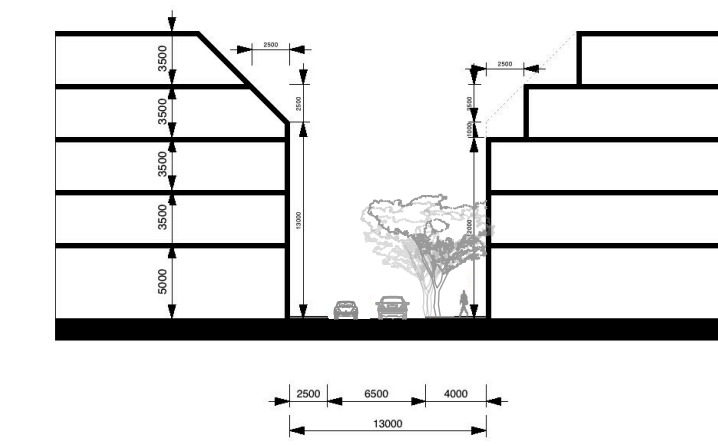
SECTION DD SCALE 1:500
