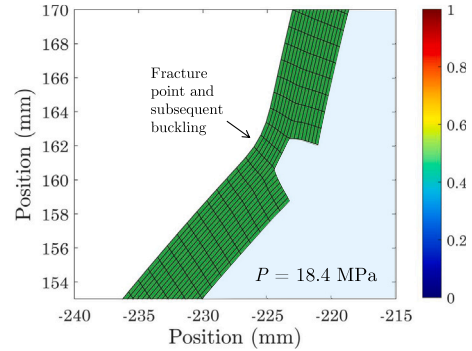
(d) Zoomed failure regions in the bottom 0° ply at 18.4 MPa.
