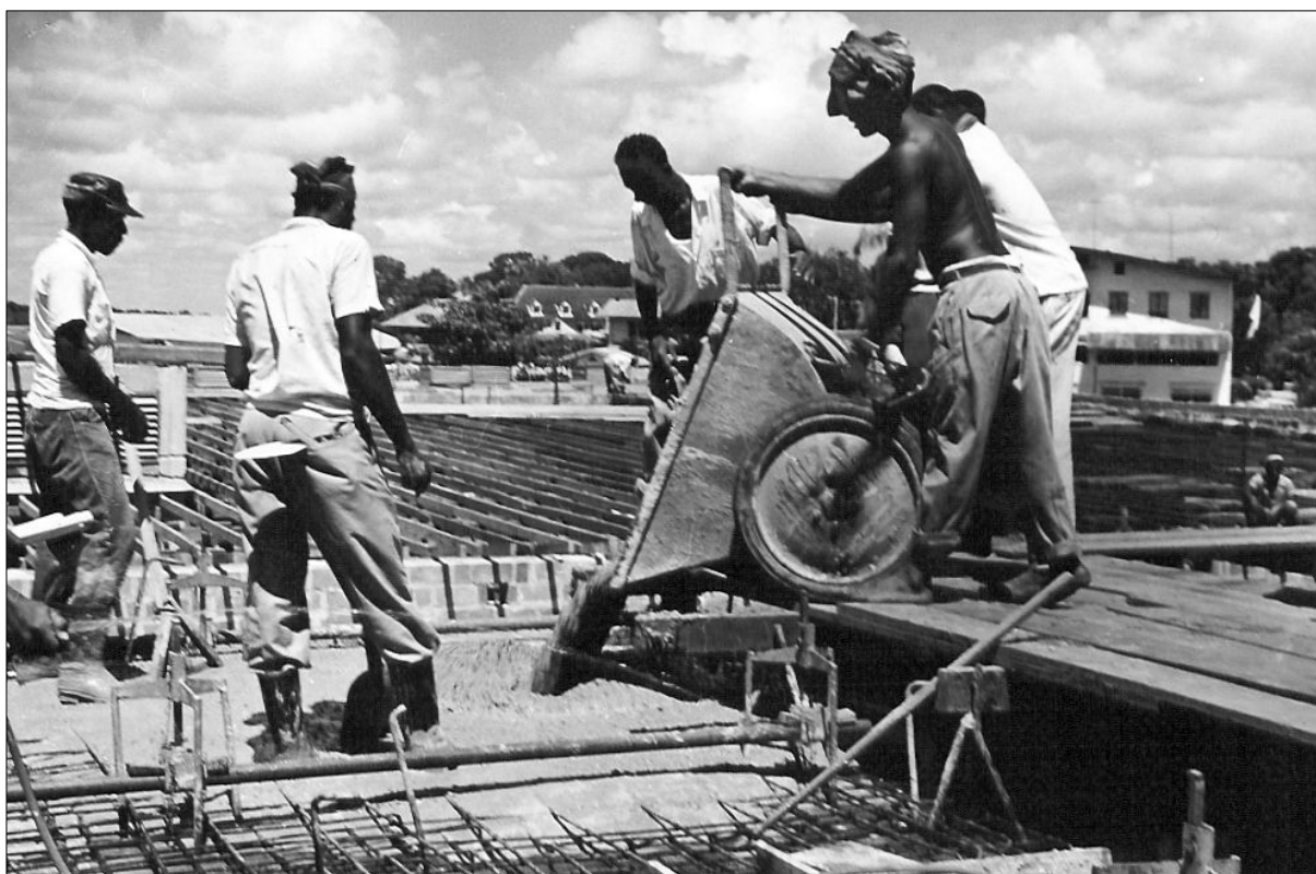
Beton storten op de vloer van de 2 e verdieping van de hotelvleugel
