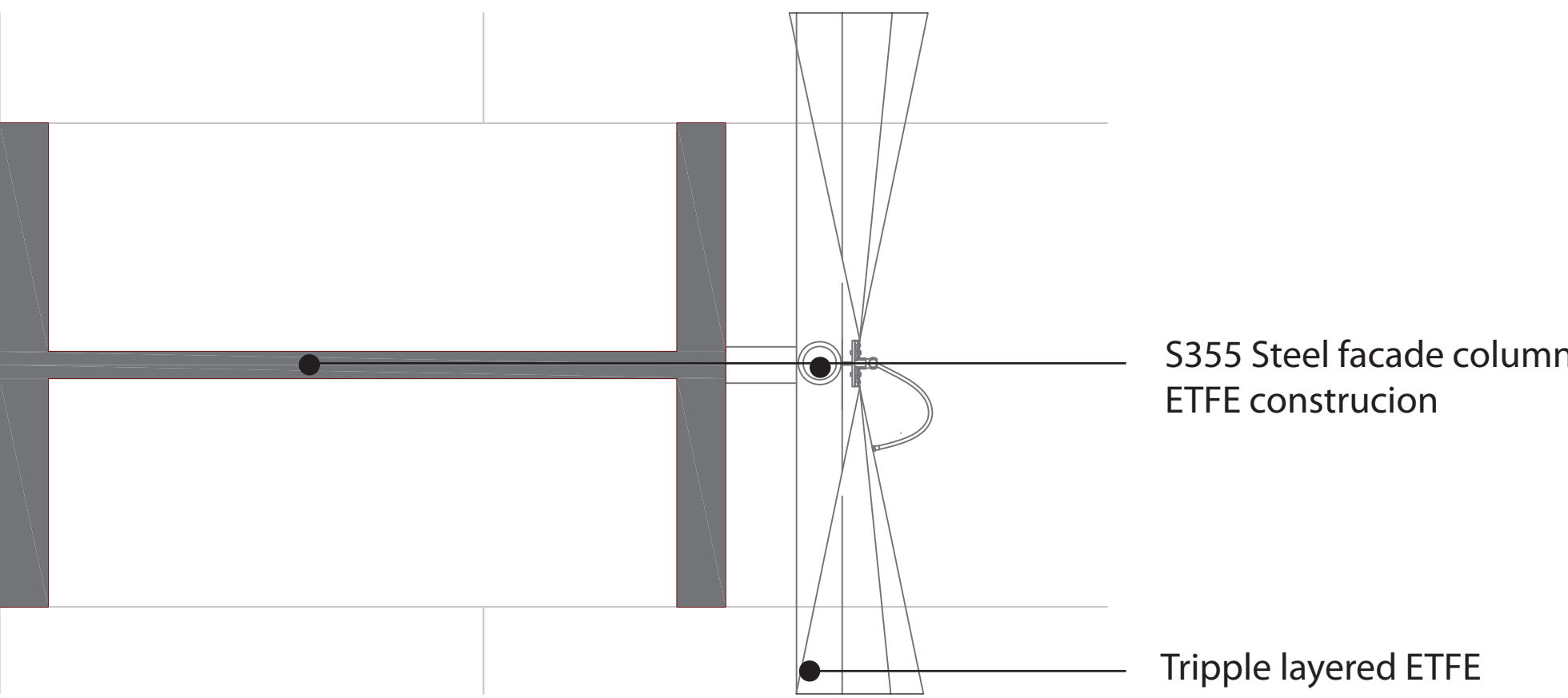
Detail 3 ETFE - ETFE
