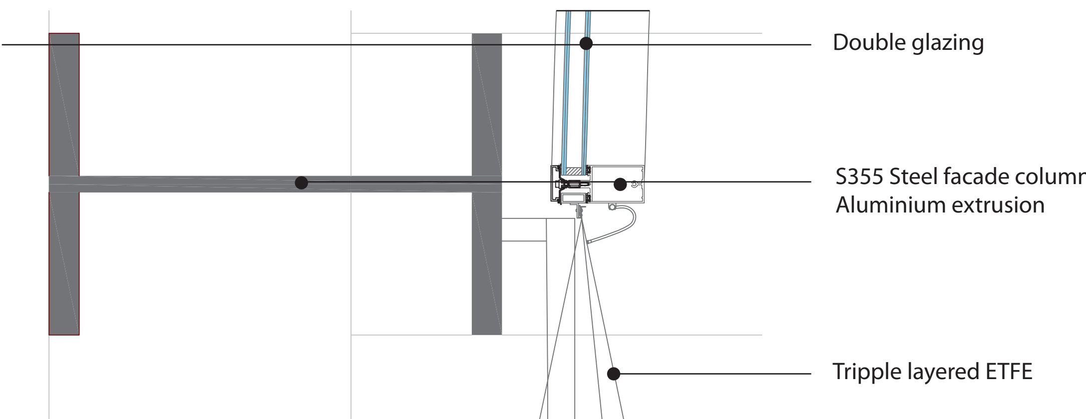
Detail 3 ETFE - ETFE
