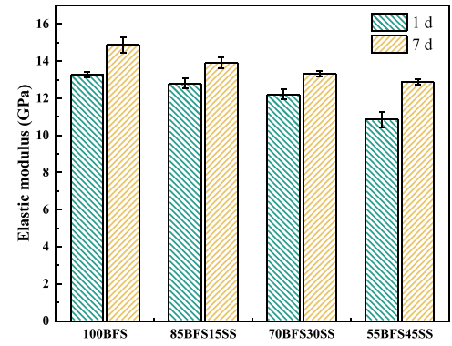
Fig. 16. Elastic modulus of AAS-SS pastes.
