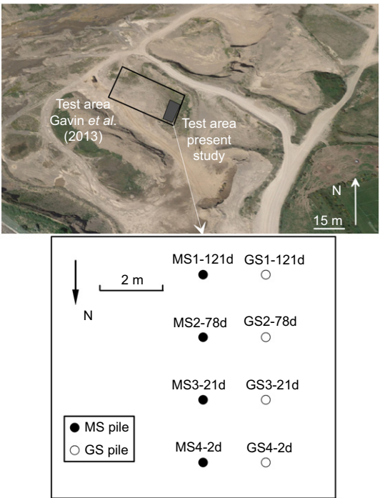
Fig. 7. Blessington site layout
