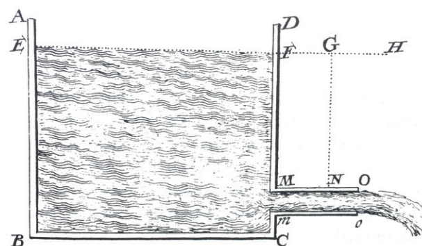
Figuur 6 Een leeglopend vat.
