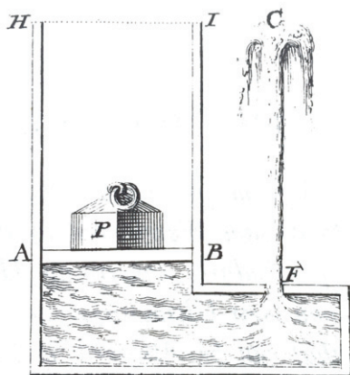
Figuur 2 Druk, snelheid en hoogte van een straal zijn equivalent.
