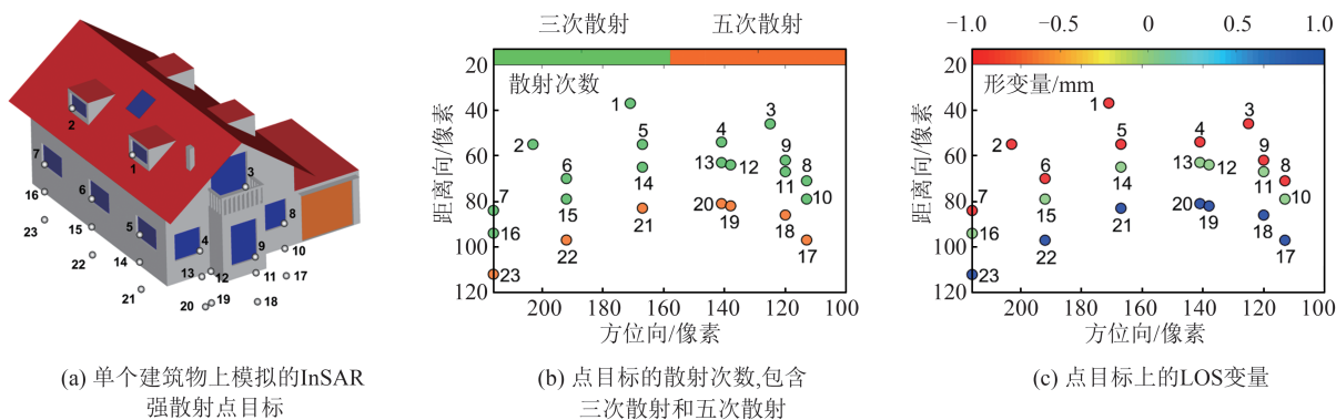
图4 文献[160]模拟单个建筑物下沉事件所探测的InSAR相干点位置、散射次数及其沿着LOS方向形变量
