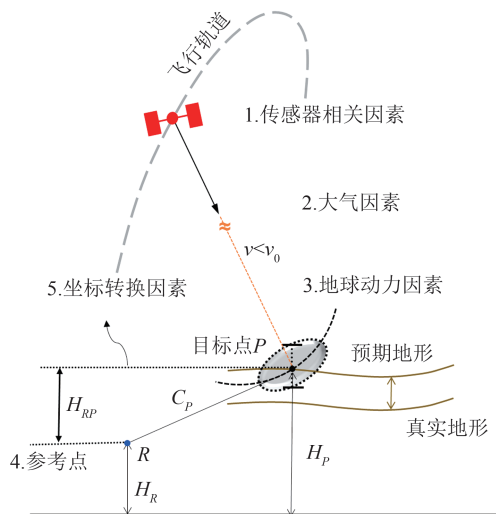
图 3 InSAR 相干点定位误差示意图
