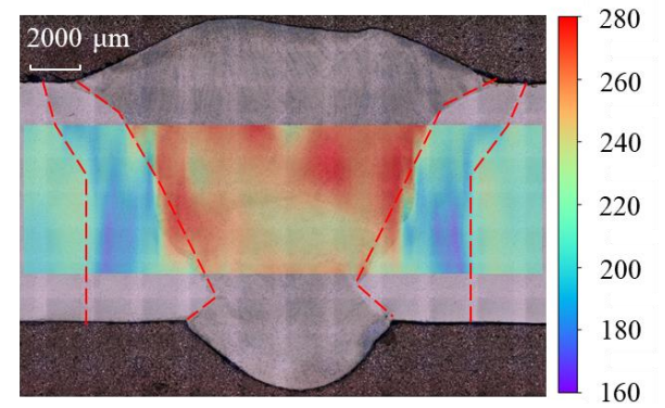
b) S500 weld zone
