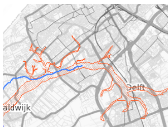
ILLUSTRATIE 5.37 De kaart toont de in de ondergrond aanwezige 'Gantelzanden' (oranje) met aan het einde de locatie van de stad Delft en de loop van de huidige Gantel (voormalige kreek).
