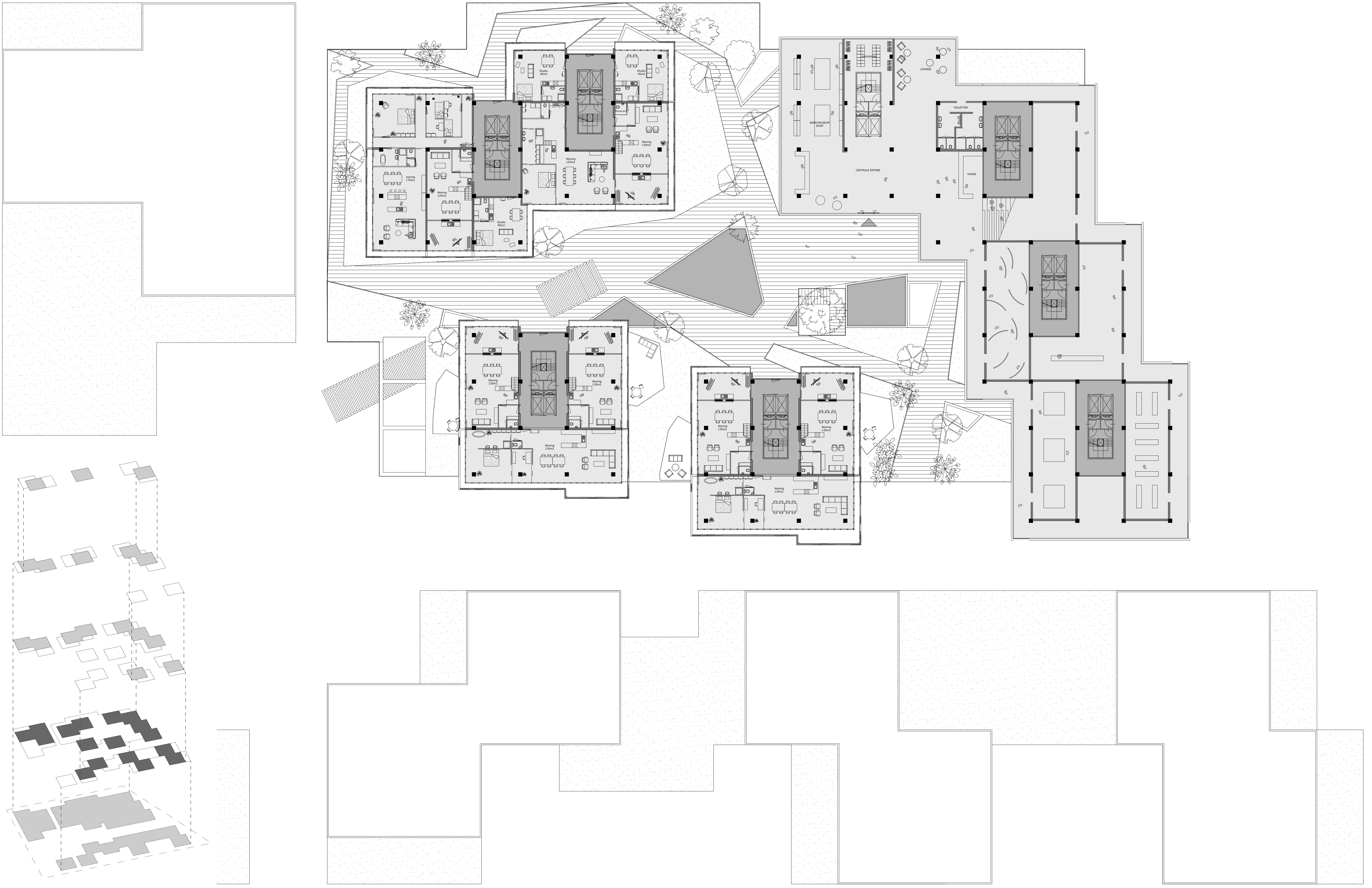
Plattegrond verhoogd maaiveld 1:200 +20.000
