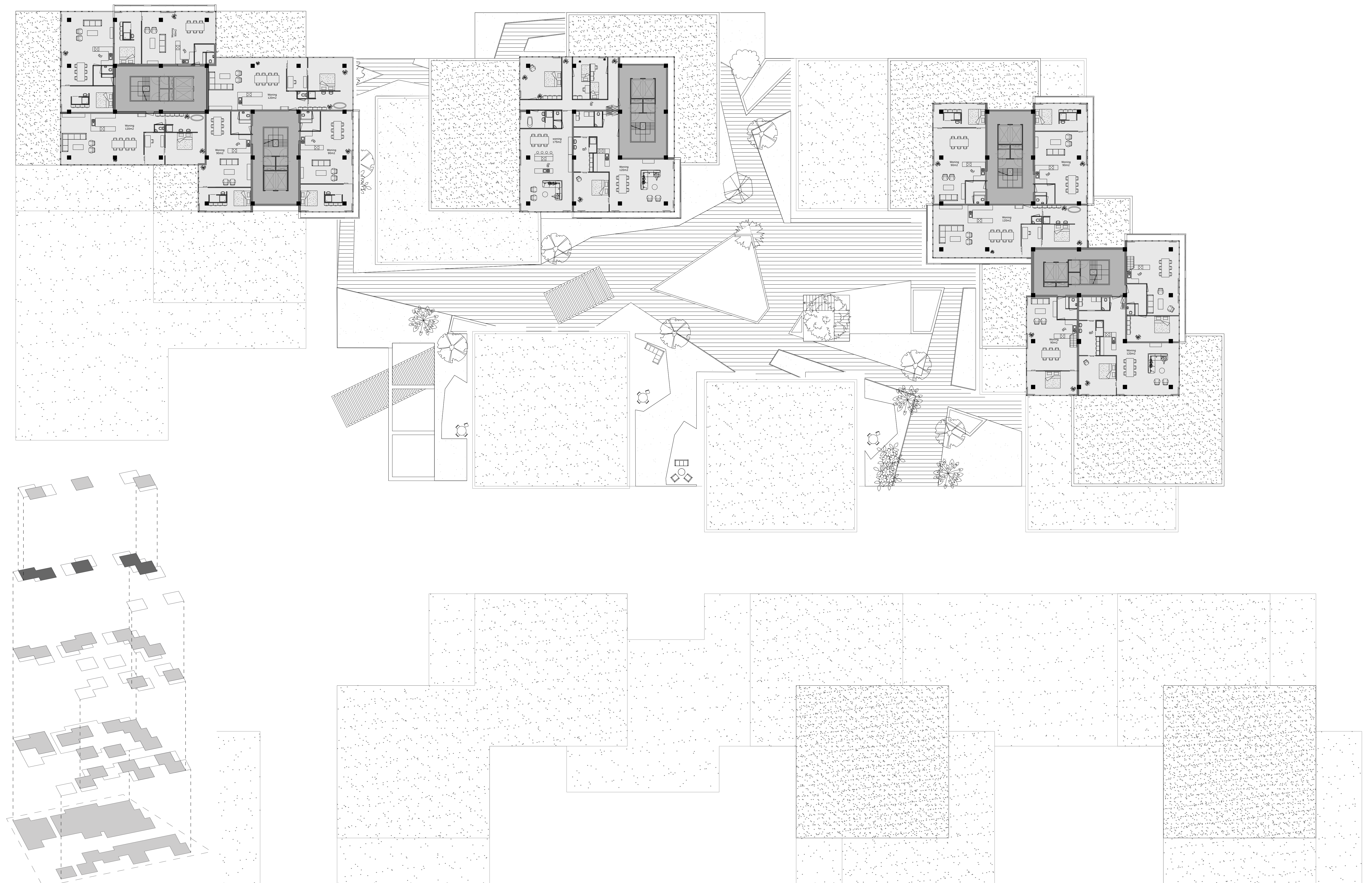
Plattegrond Verdieping 1:200 +56.400
