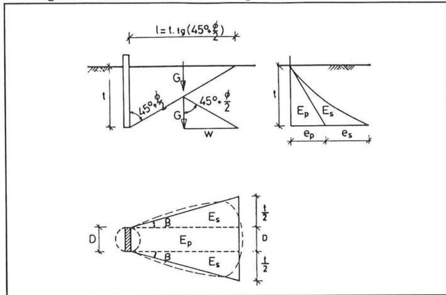
Afbeelding 48, schematisatie volgens Blum.
