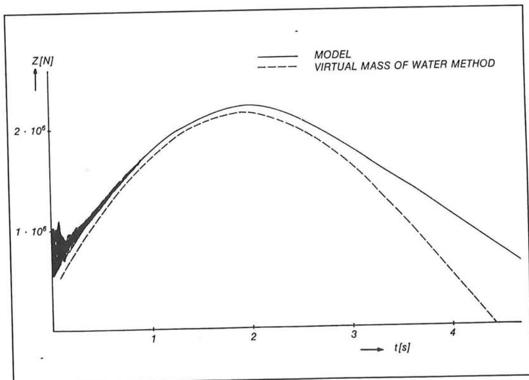
Afbeelding 3, botskracht [22].
