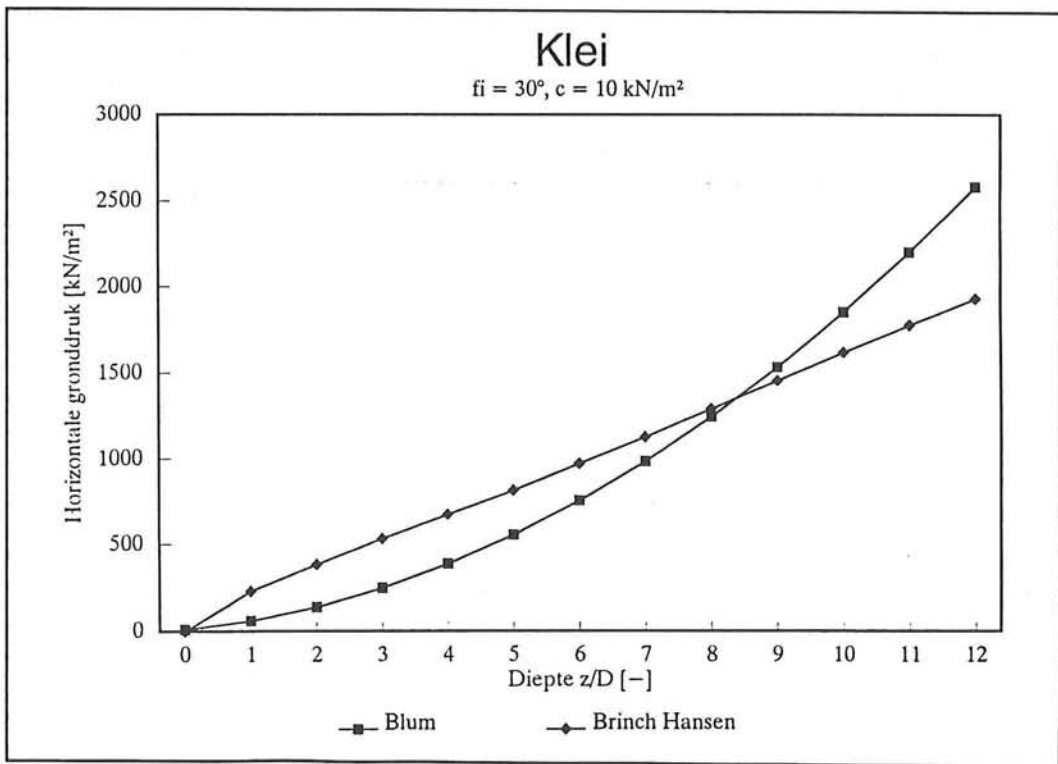
Afbeelding 25, klei.
