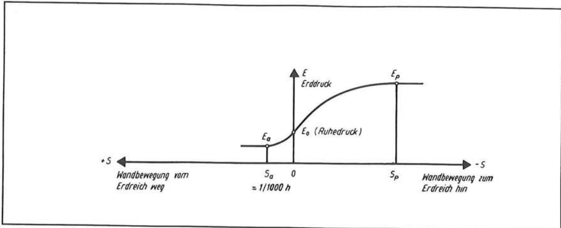
Afbeelding 20, veer karakteristiek.
