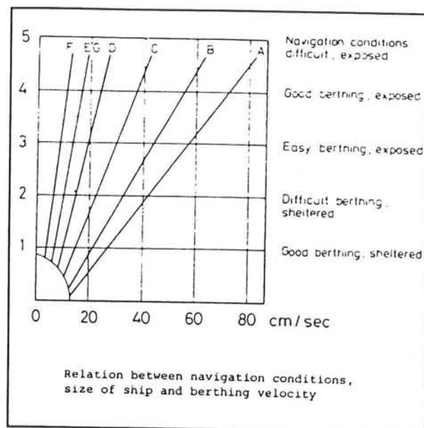
Afbeelding 7, afmeersnelheid.
