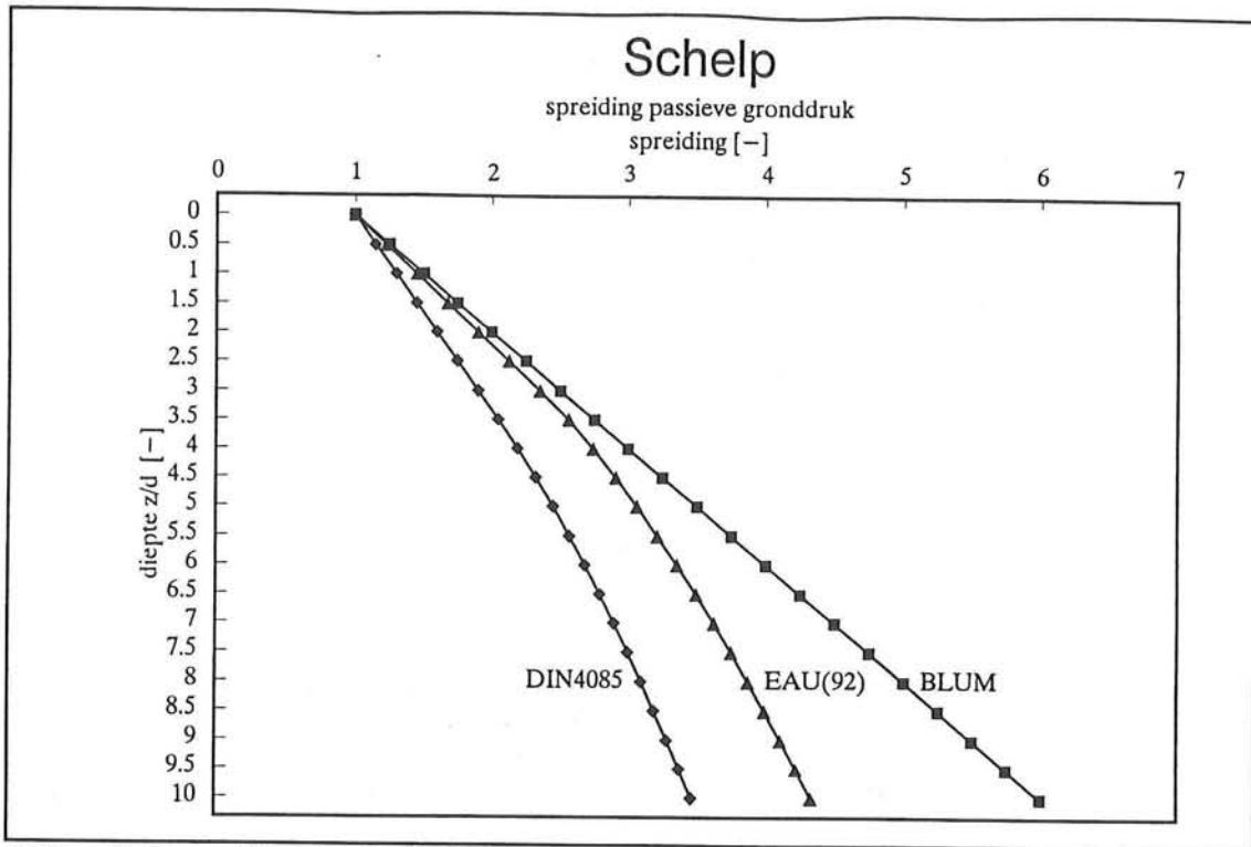
Afbeelding 19, schelffactoren.
