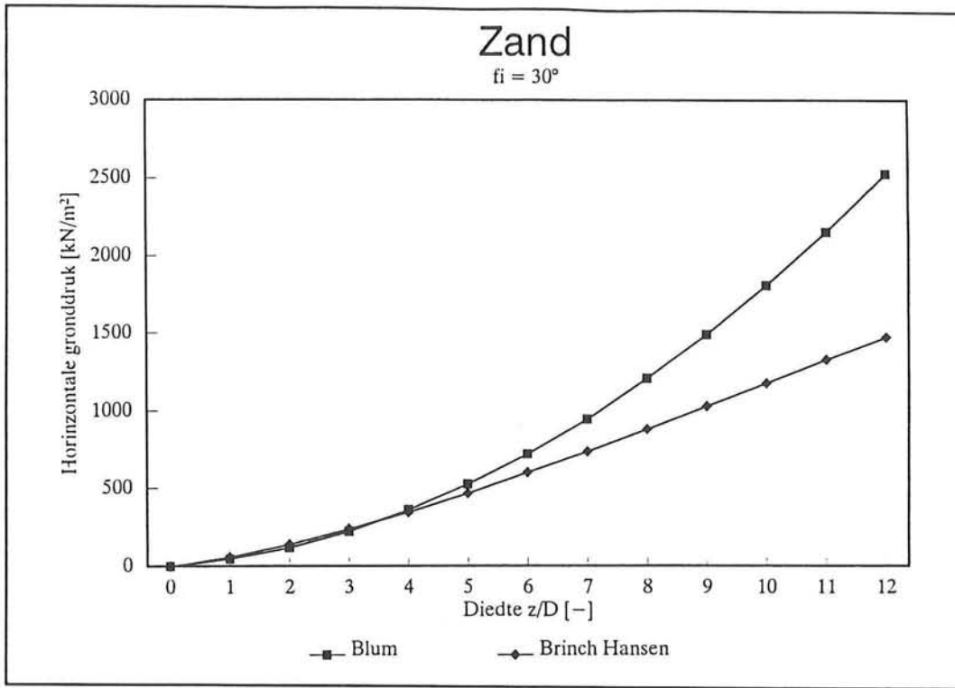
Afbeelding 24, zand.
