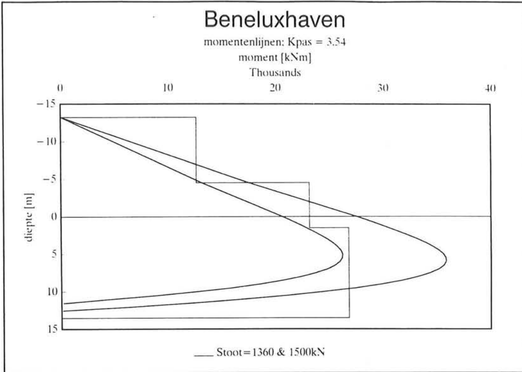
Afbeelding 38, Blum.
