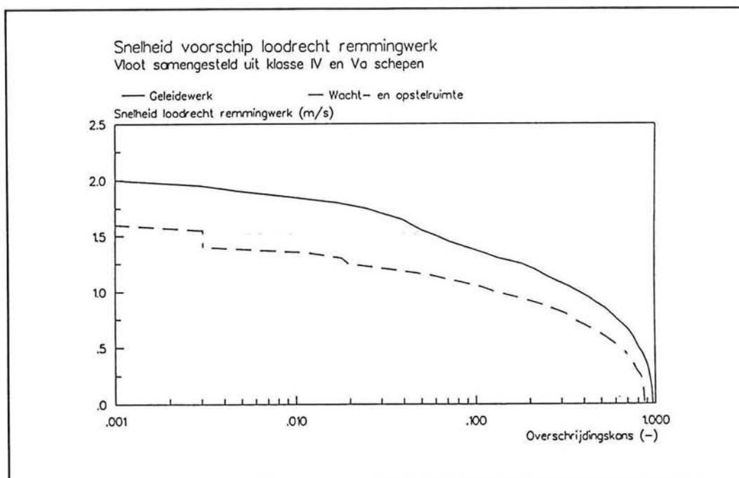
Afbeelding 9, overschrijdingskromme.
