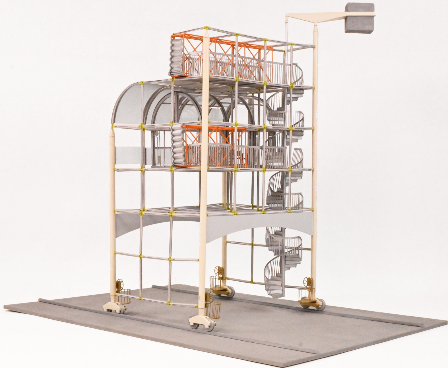
Maquette Schaal 1:20
