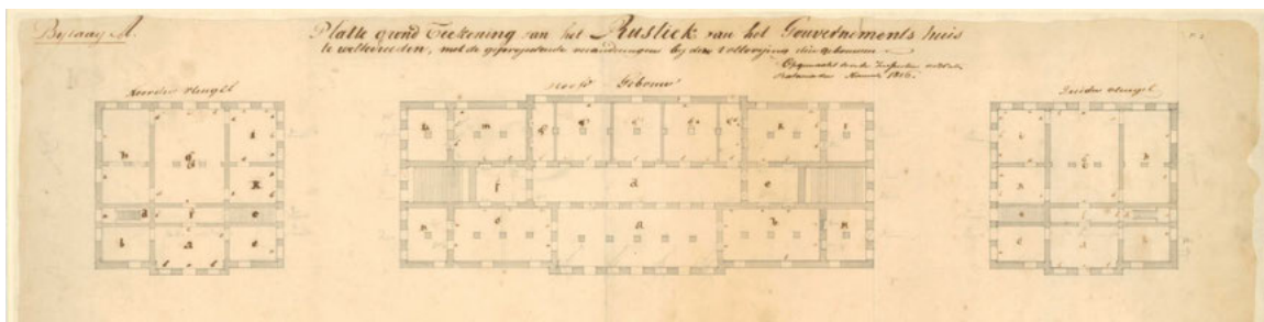
Ilustrasi 4: Gambar asli denah lantai dasar bangunan utama dan dua bangunan sayap dari Gedung Cagar Budaya Kementerian Keuangan di Weltevreden.
