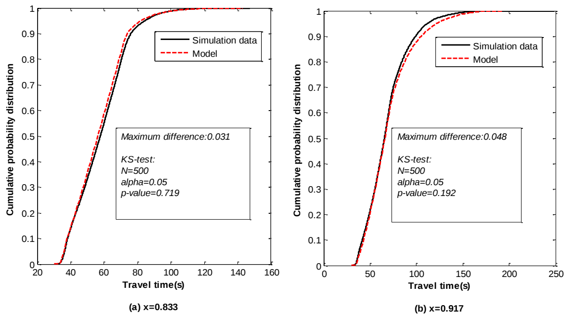
Figure 15 Kolmogorov-Smirnov test
