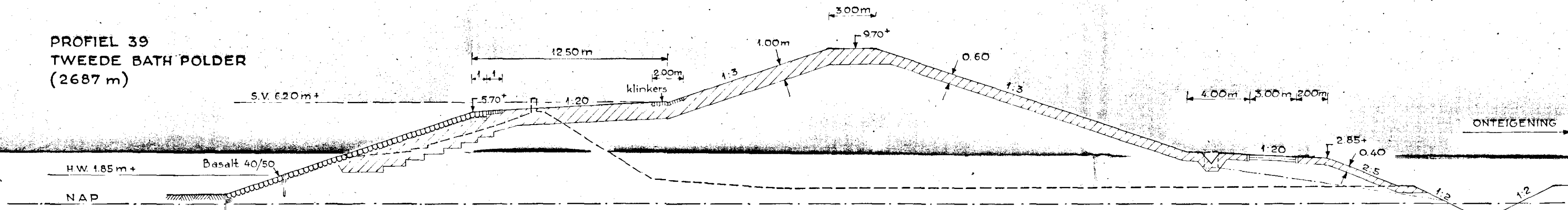
PROFIEL 40 TWEDE BATH POLDER (1536 m)
