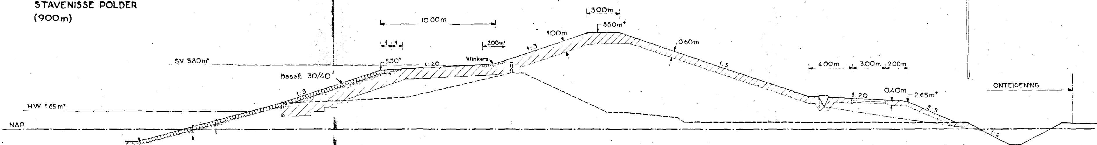
PROFIEL 66 MARGARETHA POLDER (500m)
