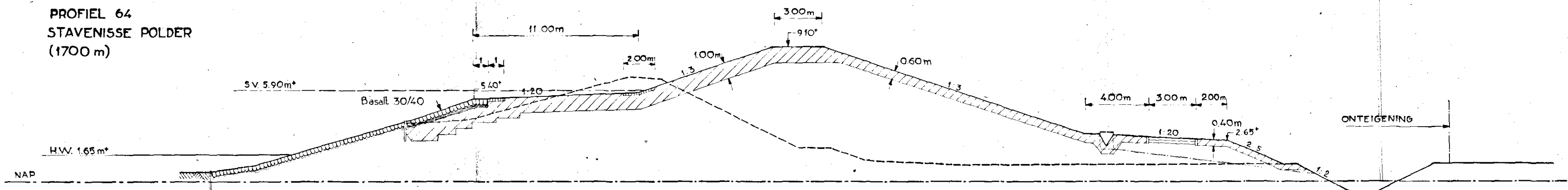
PROFIEL 65 STAVENISSE POLDER (900m)
