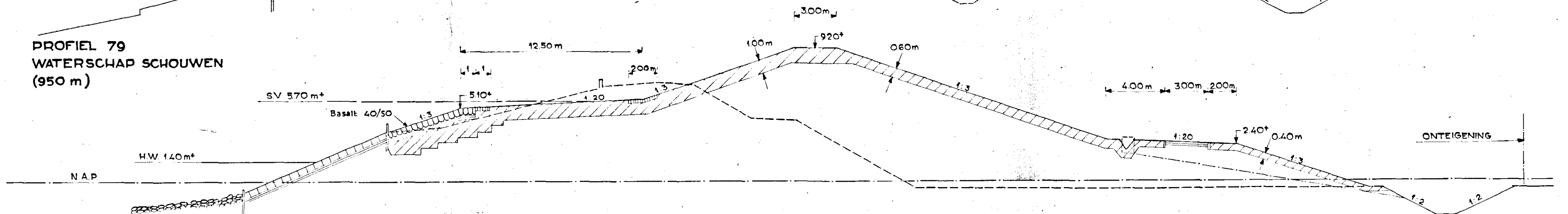
PROFIEL 80 WATERSCHAP SCHOUWEN (1575 m)
