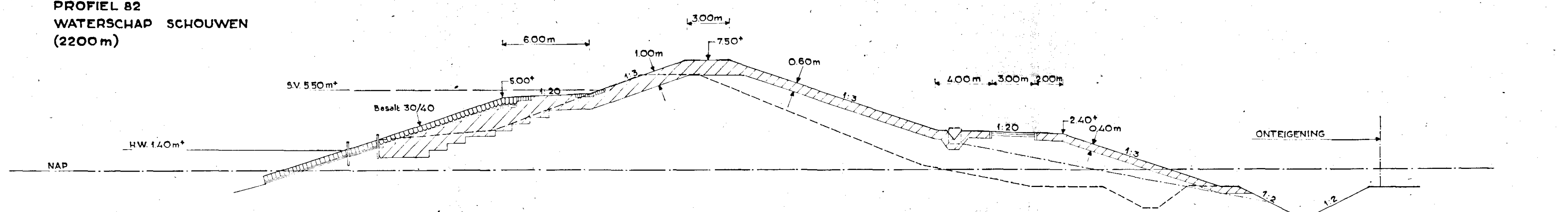
PROFIEL 83 WATERSCHAP SCHOUWEN (475 m)
