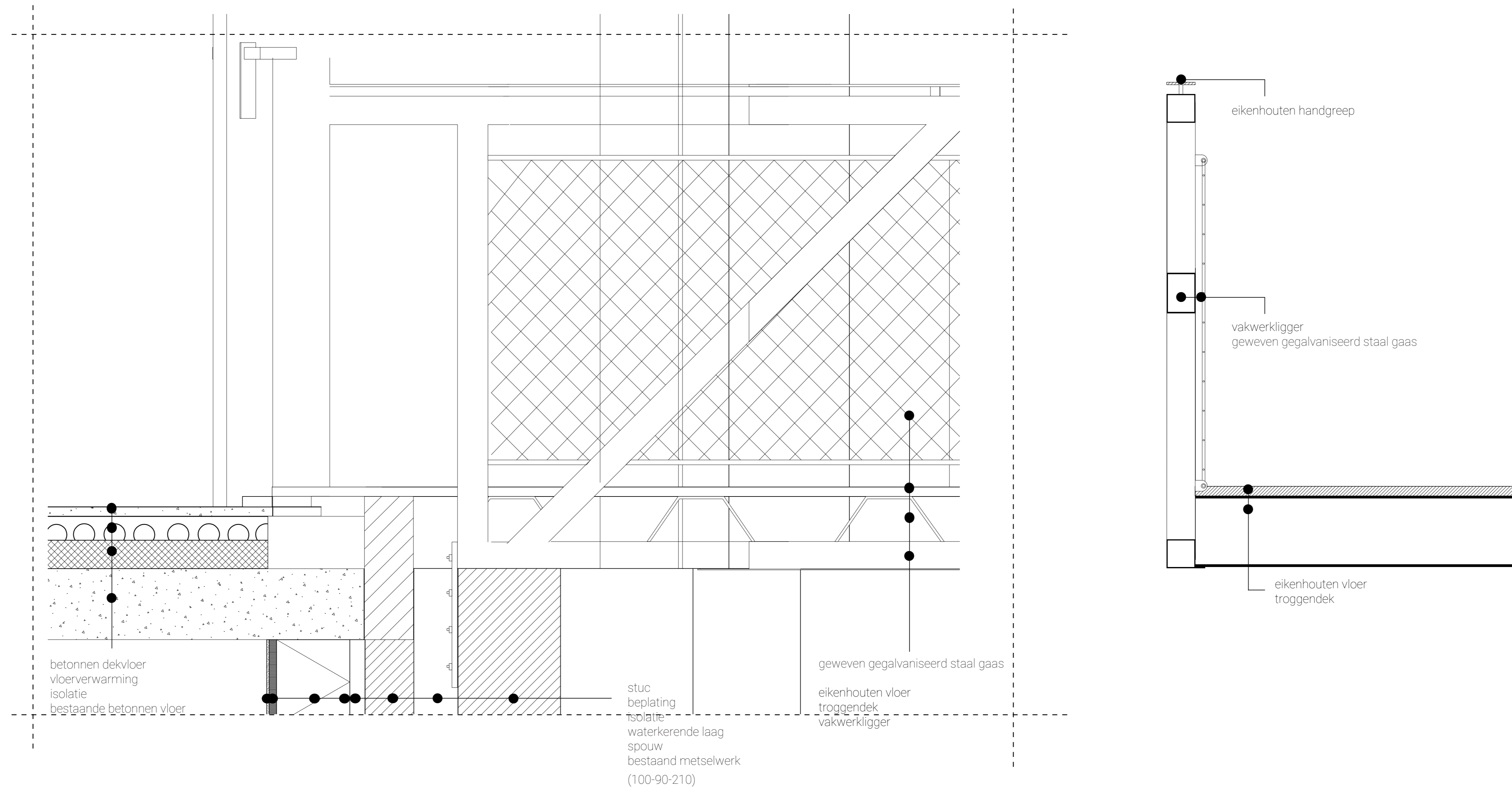
Details loopbrug 1:5
