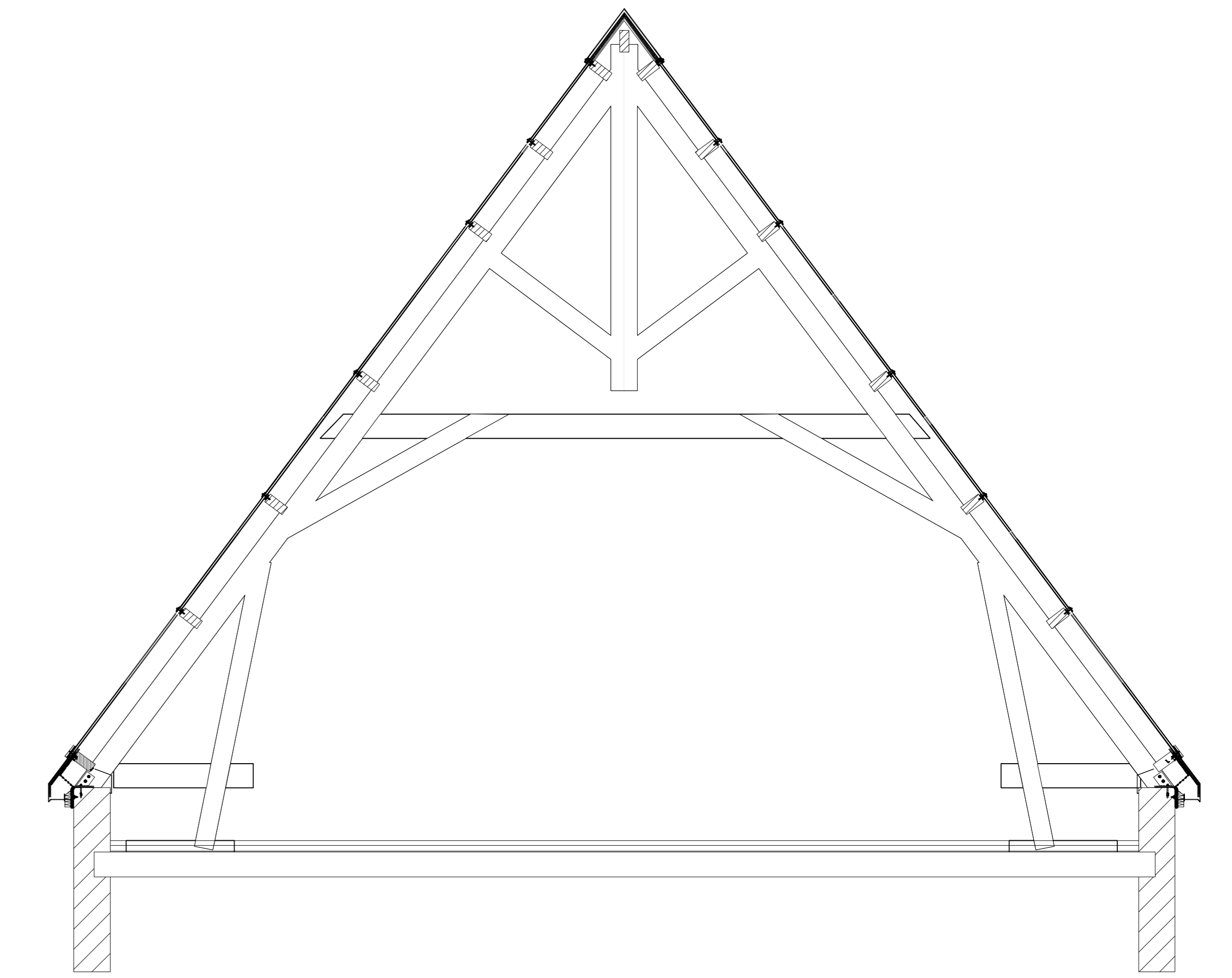
dakkas 1:50
