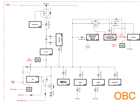
Fig. 8. OBC Block Diagram.
