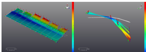
(d) Mode 7 [30.7 Hz]
