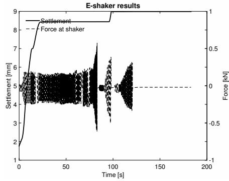
(d) Force at shaker Test 60
