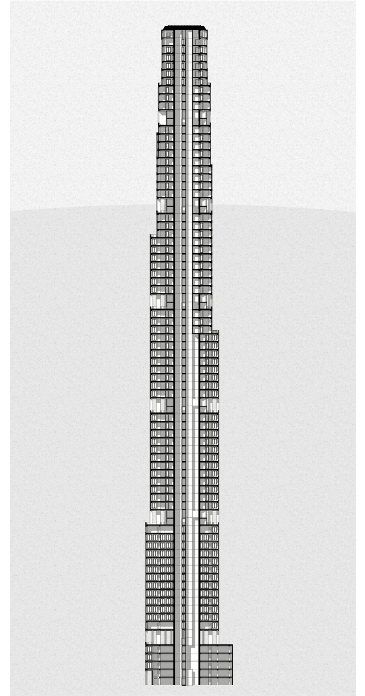
Section B: Longitudinal
